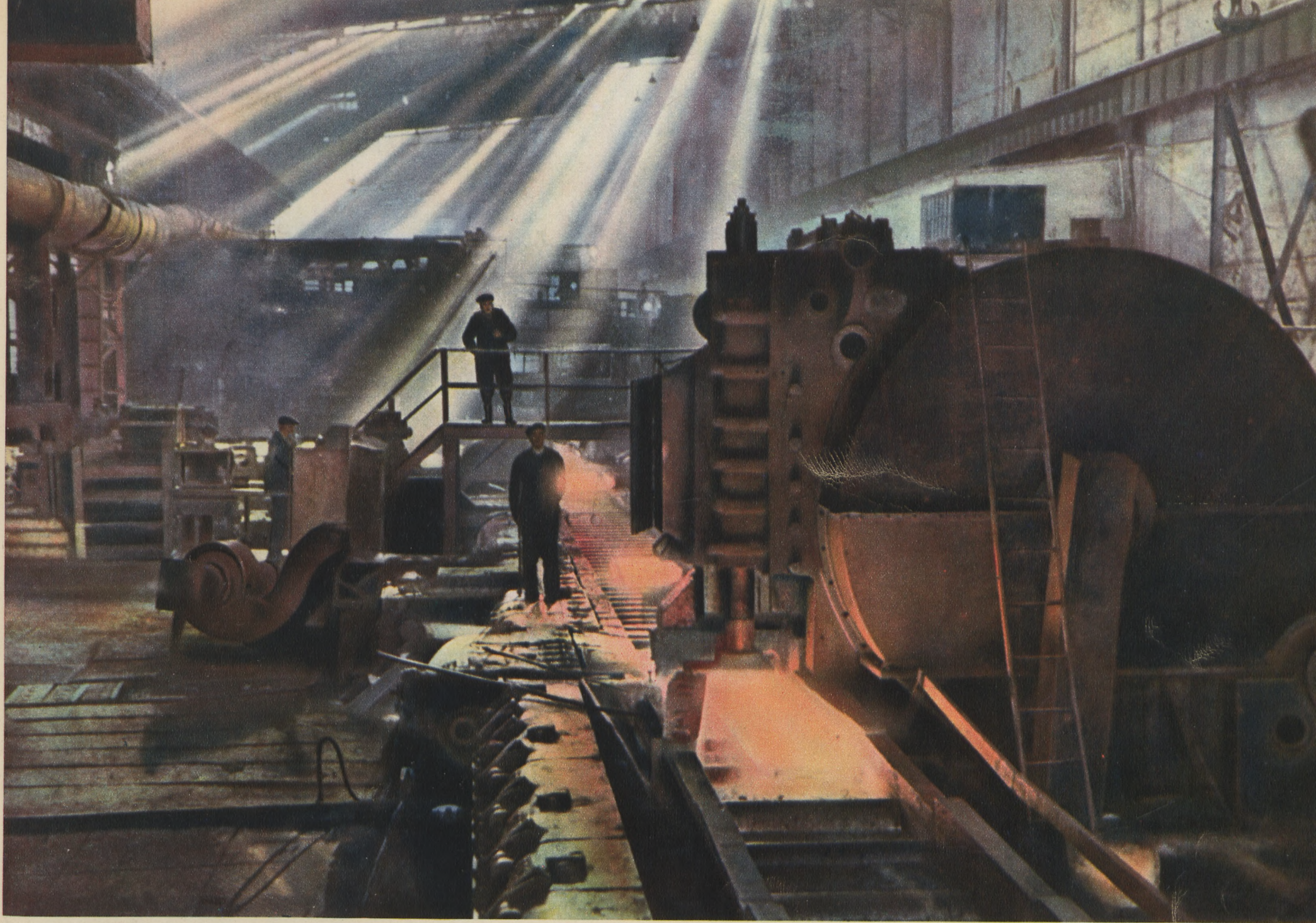
В цехе блюминга. Ножницы прокатного стана „1100” обрезают стальной слиток до заданных размеров.
