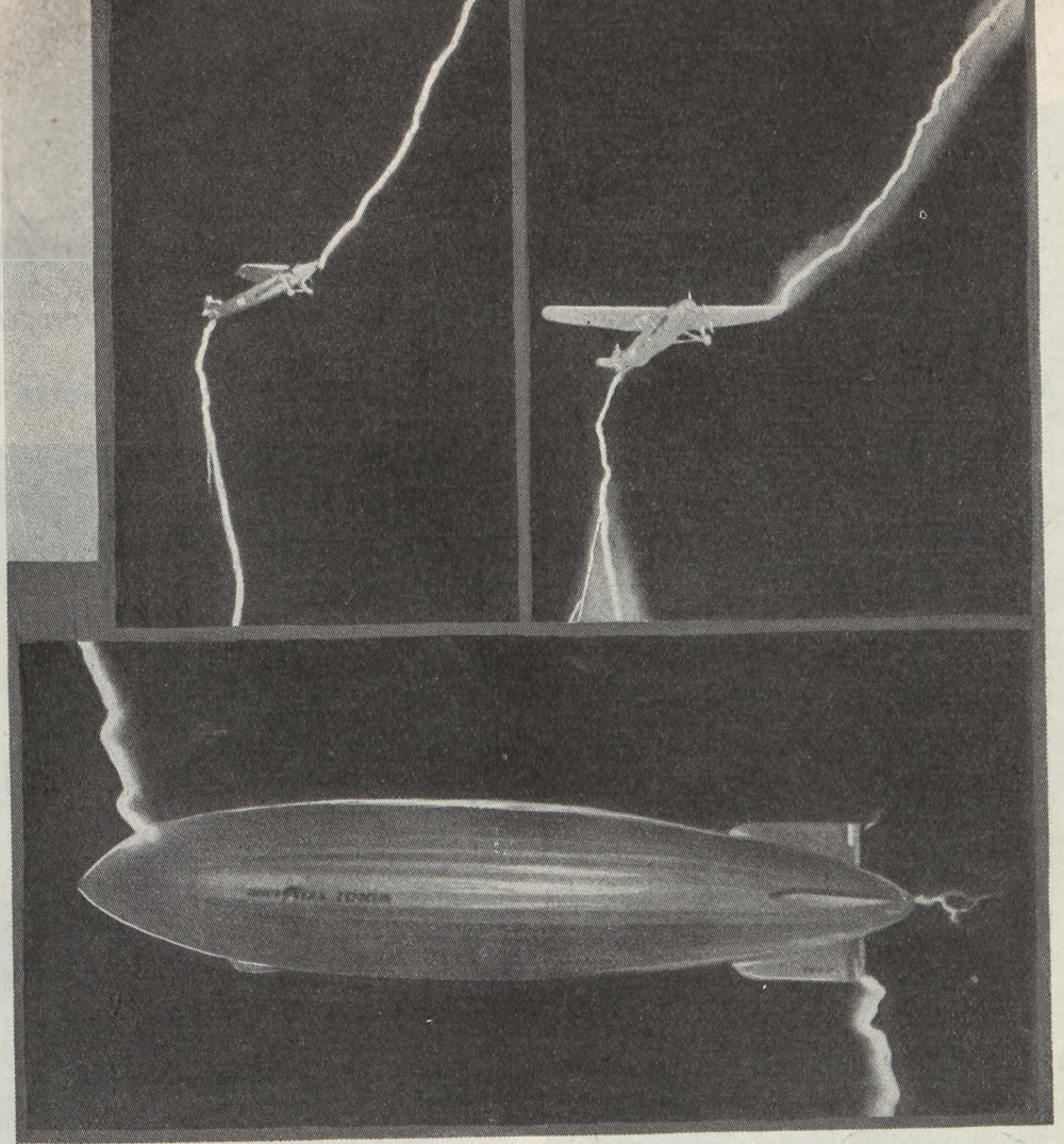
Искусственная молнія проходитъ сквозь модель летательнаго аппарата, не причиняя ему вреда.
