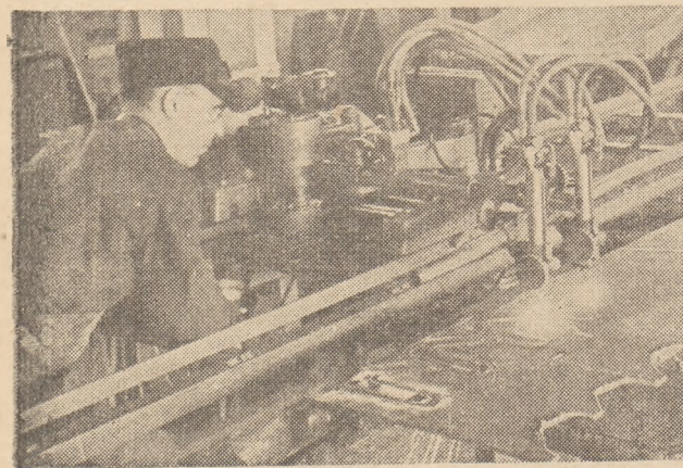
Cięcie blach stalowych płomieniem.
