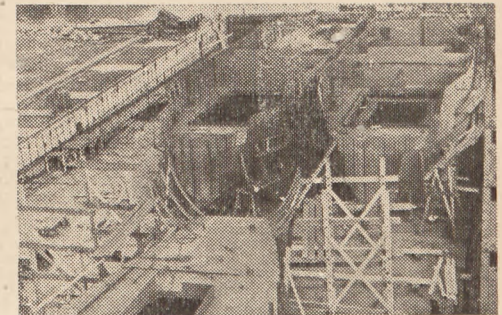
Rośnie nasza flota. Oto kadłuby trzech z serii pięciu drobnalcowców motorowych po 650 DWT, budowanych na jednej z polskich stoczni. Jak widać, piece są już znacznie zaawansowane.
