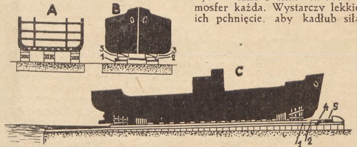
Rysunek A przedstawia statek w budowie. Widoczne są trzy rzędy kozłów, na których konstruuje się kadłub. Rysunki B i C przedstawiają statek przygotowany do wodowania: prowadnice oznaczone są cyfrą — 1, płozy — 2, kliny — 3, stoper — 4 a prasy hydrauliczne — 5.
