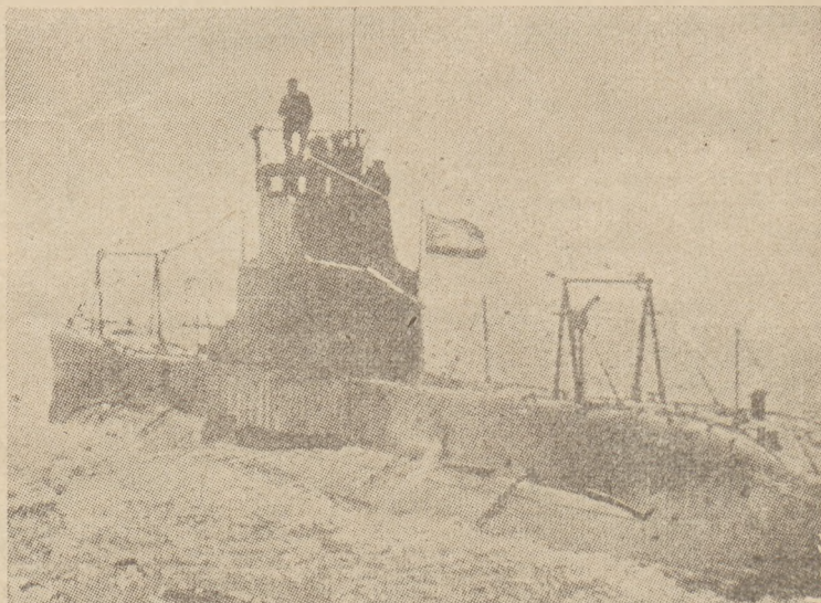
Radziecki okręt podwodny klasy „Malutka“. Jednostki z tej serii zdobyły powszechne uznanie swymi doskonałymi zaletami morskimi i bojowymi.
