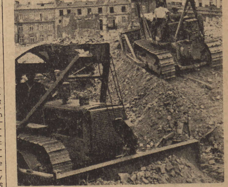
1 sierpnia br. przystąpiono do budowy pierwszego odcinka Marszałkowskiej Dzielnicy Mieszkaniowej (MDM) w Warszawie. Na zdjęciu zmechanizowane odgruzowanie terenu przy ul. Marszałkowskiej. Wielki spychacz „Staliniest”, produkcji radzieckiej, w ciągu dnia pracy usuwa od 600 do 700 m sześci. gruzu. Foto AR
