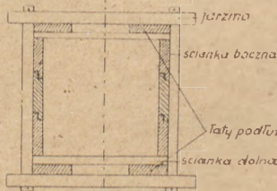
Lżak przekrój a - b
