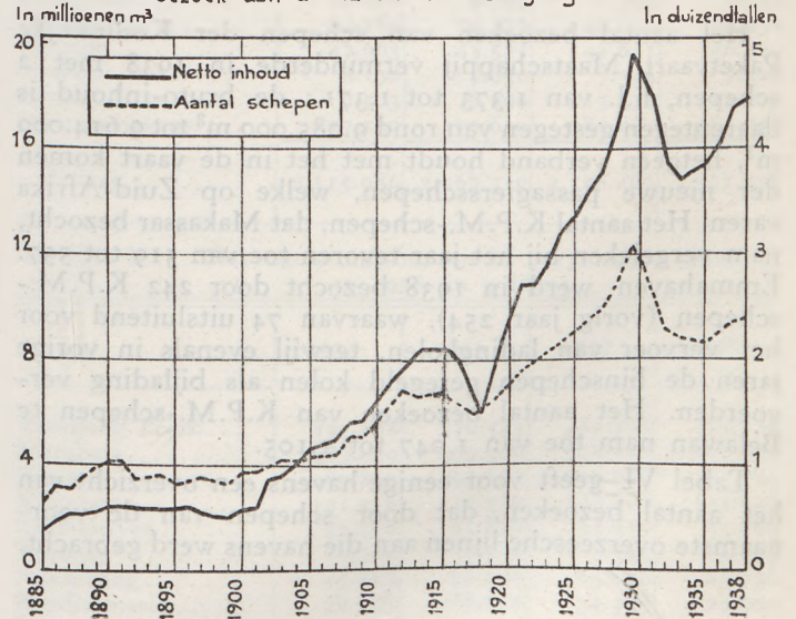
GRAFIEK 3 Aantal schepen en netto inhoud van het scheepsbezoek aan de haven van Tandjong Priok.
