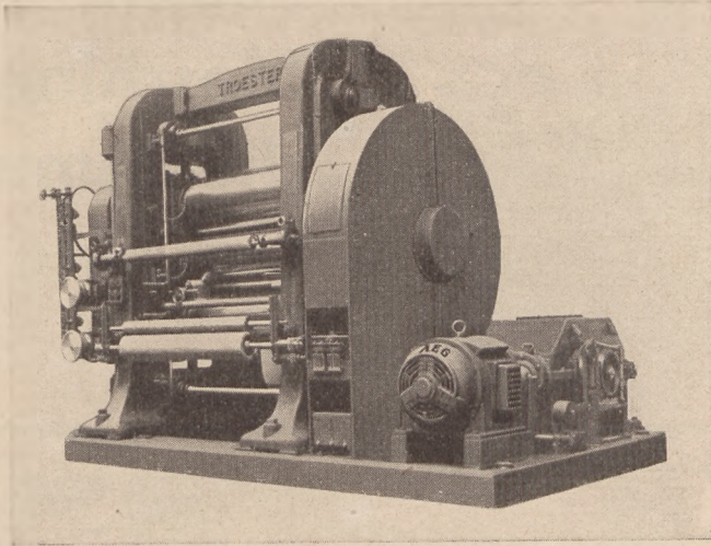
Kalander mit vierfach polumschaltbarem Ds-Motor 1500/1000/750/500 U/min bei 58/48/37/30 kW
