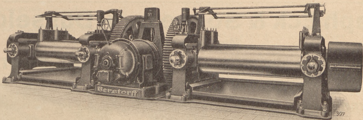
Gruppenantrieb
