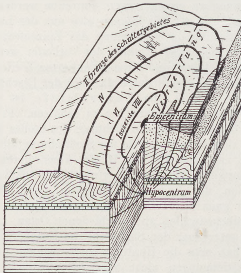
Fig. 187 Modell zur Veranschaulichung der Entstehung eines tektonischen Erdbebens und der wichtigsten seismologischen Begriffe (nach A. Sieberg). Die römischen Zahlen geben die Stärke des Bebens nach der zwölfstufigen Skala.
