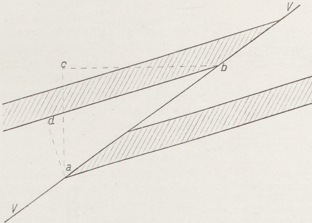
Fig. 124 Überschiebung auf einer Wechselfläche V-V . a-b ist die flache, a-c die seigere, a-d die wirkliche Sprunghöhe.
