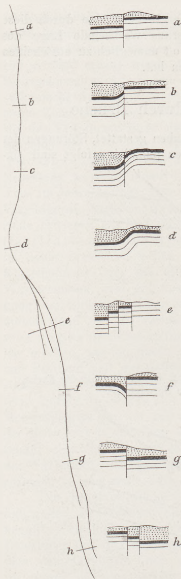
Fig. 125 Veränderung einer Verwerfung in ihrer Erstreckung: a ) einfache Verwerfung, b ) Schleppung des abgesunkenen Flügels, c ) Schleppung beider Flügel, d ) Flexur, e ) treppenförmiges Absinken an divergierenden Spalten, f ) Schleppung des Liegendflügels durch nachträgliches Absinken des Hangendflügels oder starkes Absinken an der Bruchlinie, g ) einfache Verwerfung des Gegenflügels u. h ) treppenförmiges Absinken an vikariierenden Spalten in entgegengesetzter Richtung (nach F. Löwl)
