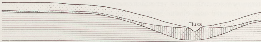
Fig. 287 Verlauf des Grundwassers in einer Hügellandschaft. Undurchlässiges Gestein ist horizontal schraffiert, durchlässiges Material punktiert, Grundwasserschicht senkrecht schraffiert. Das Wasser strömt dem Flusse zu.
