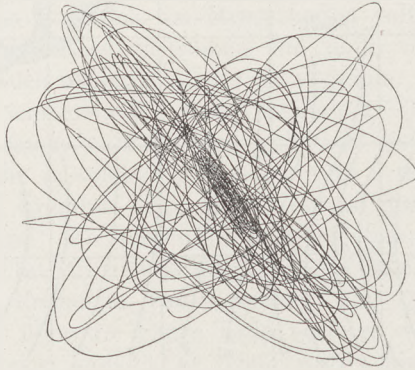
Fig. 209 Diagramm des Philippinenbebens 15. Dezember 1901 (nach F. de Montessus de Ballore)
