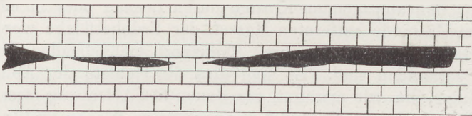
Fig. 362 Auskeilen, Wiederaufsetzen und Abschneiden einer Schicht, linsenförmige Einlagerung
