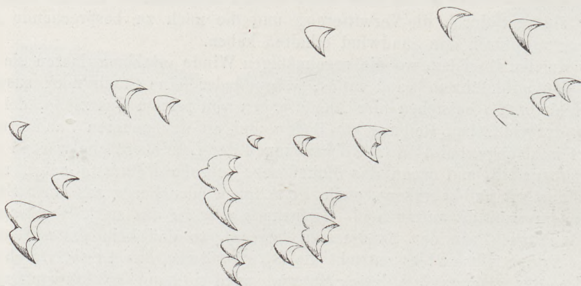
Fig. 349 Grundriß neu entstandener Barchane bei Buchara (nach J. Walther)
