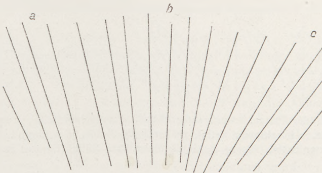
Fig. 145 Fächerförmiger Schichtbau; die bei a monoklinal aufgerichteten Schichten stehen bei b seiger und liegen bei c überkippt.
