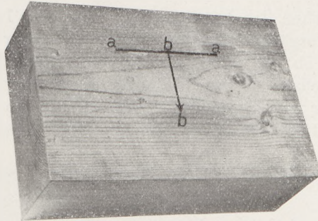
Fig. 117 Streichen ( a-a ) und Fallen ( b-b ) einer Schichtfläche
