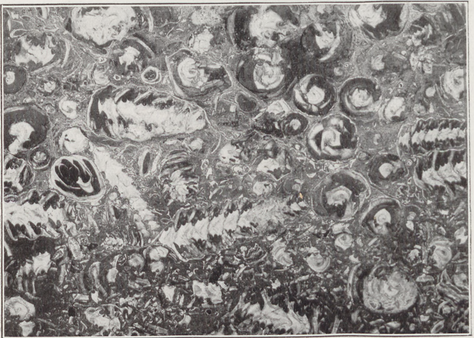
Fig. 467 Nerineenkalk, obere Kreide, Sengsengebirge. Die Gehäuse sind zum Teil mit Sediment, zum Teil mit weißem Kalkspat erfüllt.
