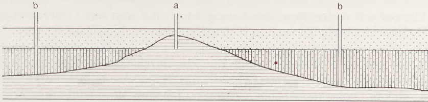
Fig. 286 Aus dem wasserführenden (senkrecht schraffierten) Sande (punktiert) ragt eine Erhebung von undurchlässigem Gestein (horizontal schraffiert) auf. Brunnen a gibt kein Wasser, die Brunnen b, b sind ergiebig.
