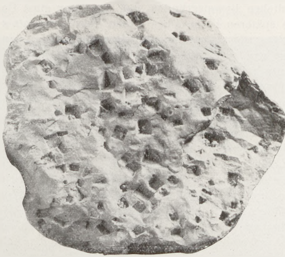
Fig. 426 Abdrücke von Salzkristallwürfeln auf der Unterseite einer Schicht
