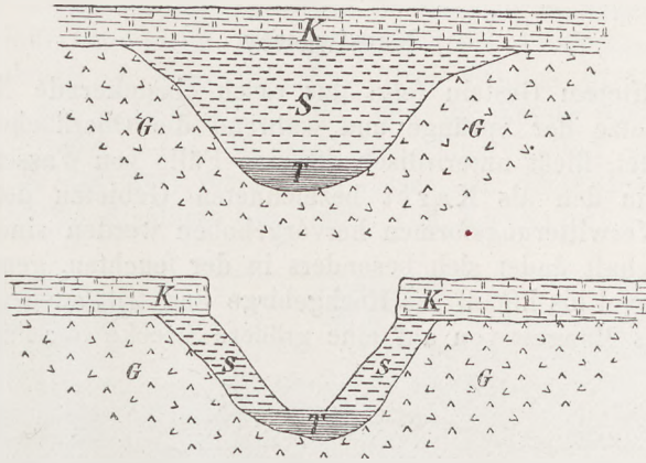
Fig. 290, 291 Anekathäretische Erosion. G Granit, T Tegel, S Sand, K Kalkstein
