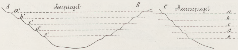
Fig. 278 Der Zusammenhang der Ausbildung der Terrassen bei Wien (A) mit der der relativ gleich hohen am Ausgange des Eisernen Tores (B—C). a-e , a'-e' Wasserstände
