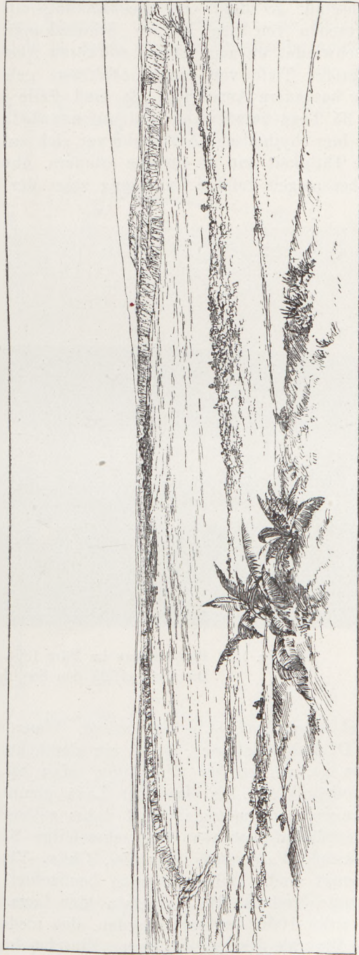
Fig. 99 Kilauea-Krater, von Volcano house gesehen (nach C. E. Dutton).
