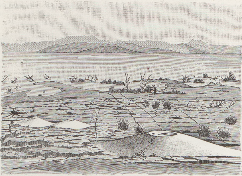
Fig. 201 Gesunkener Strand mit Spalten und Sandkratern, achäisches Erdbeben 26. Dezember 1861 (nach J. Schmidt aus R. Hörnes)
