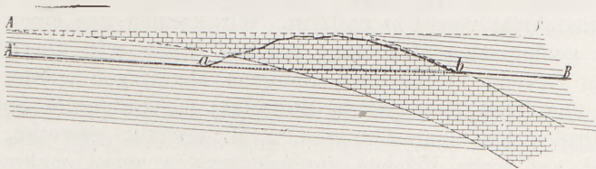
Fig. 284 Entstehung eines Durchbruchstales a b durch Abtragung des Hinterlandes und Hervortreten einer eingeschalteten widerstandsfähigen Gesteinsschicht im Relief.
