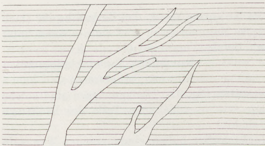
Fig. 33 Apophysen im Gestein
