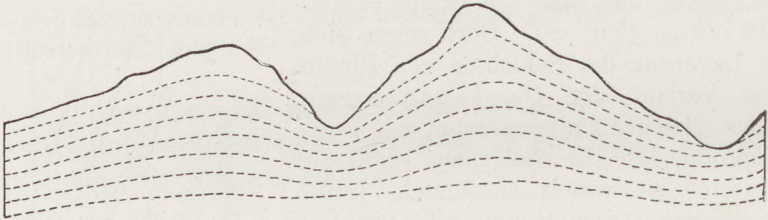
Fig. 10 Verlauf des Geoisothermen (gestrichelt), beeinflusst durch das Relief der Erdoberfläche.
