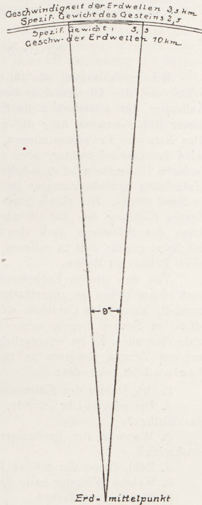
Fig. 213 Erdrinde und Erdkern in ihren relativen Maßen auf Grund der Beobachtung der Geschwindigkeit von Erdbebenwellen (nach Hobbs-Ruska)
