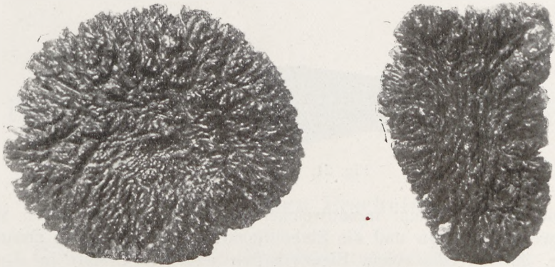
Fig. 20, 21 Moldavite mit stark skulpturierter Oberfläche
