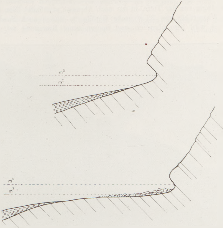
Fig. 311, 312 Ausbildung der Strandplattform mit Brandungskehle und Halde. m^1 Niedrig-, m^2 Höchstwasserstand
