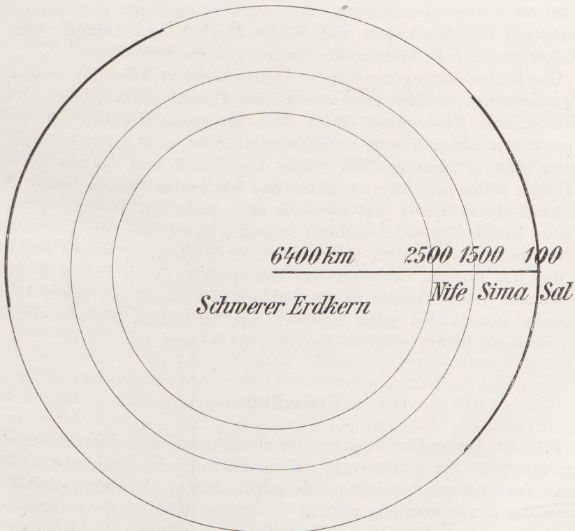
Fig. 8 Schematischer Durchschnitt durch die Erde mit den einzelnen Kugelschalen (nach E. Suess, E. Wiechert und A. Wegener)
