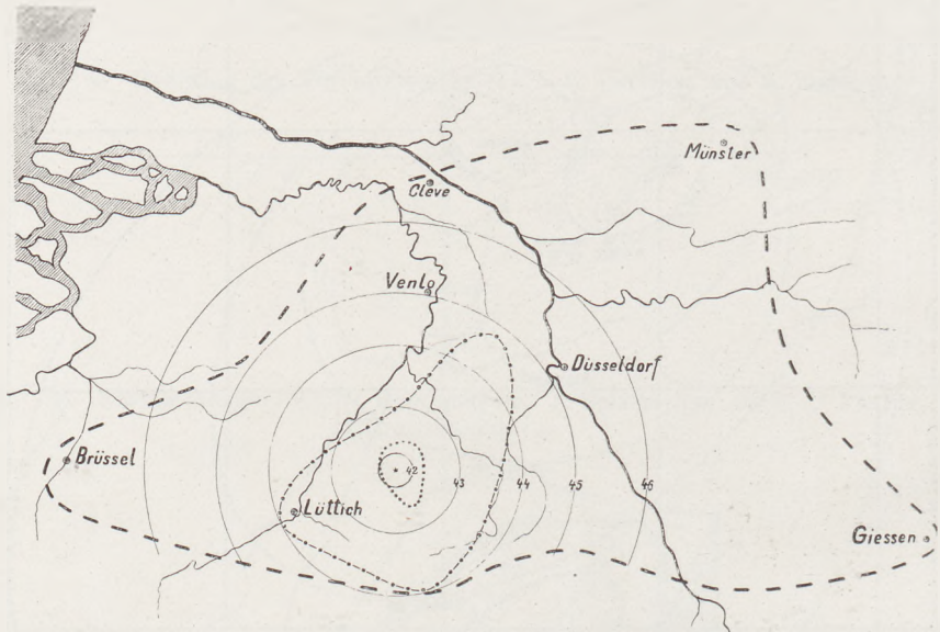
Fig. 189 Homoseismen und Isoseismen des Erdbebens von Herzogenrath am 22. Oktober 1873 (nach A. v. Lasaulx)
