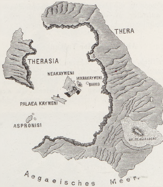
Fig. 110 Insel Santorin (nach v. Seebach)
