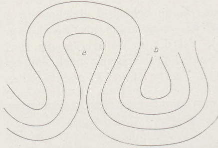
Fig. 150 a Fächersattel, b Fächermulde
