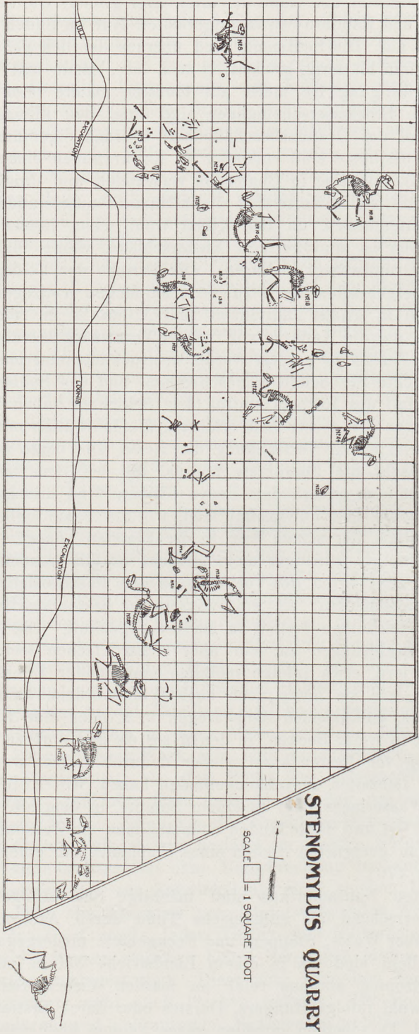
Fig. 470 Blößelegte Schichtfläche mit zahlreichen Exemplaren von Stenomylus (einer kleinen Kamelform), Miozän Nebraska (nach O. A. Peterson)
