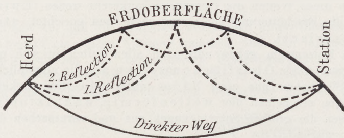
Fig. 185 Reflexion der Vorläuferwellen (nach E. Wiechert aus A. Sieberg)
