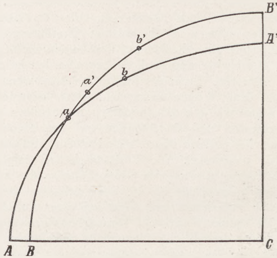
Fig. 479 Die Verschiebung der Punkte eines Meridianquadranten der Erdoberfläche beim Übergange in die inhaltsgleiche Kugel (nach A. v. Böhm). C Mittelpunkt, A (am Äquator) kommt nach B, A' (Pol) nach B'. a nach a', b nach b'.
