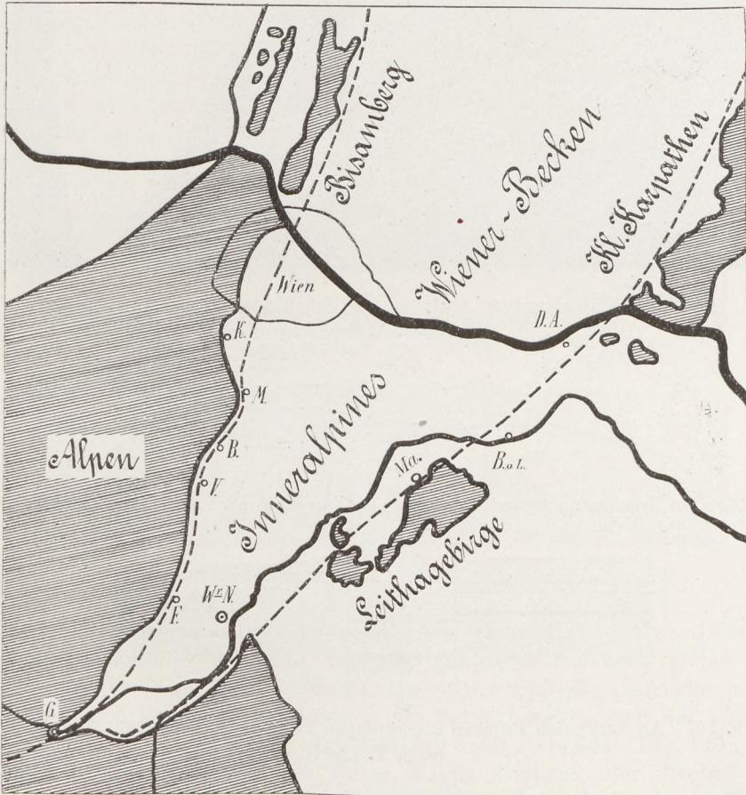
Fig. 134 Bruchfeld des Inneralpinen Beckens von Wien, das an zwei (gestrichelten) Bruchlinien abgesunken ist. K. Kalksburg, M. Mödling, B. Baden, V. Vöslau, F. Fischau, G. Gloggnitz, W. N. Wiener-Neustadt, Ma. Mannersdorf, B. a. L. Bruck an der Leitha, D. A. Deutsch-Altenburg
