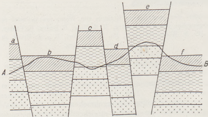
Fig. 138 Absinken und Aufpressung von Schollen an schrägen Bruchflächen
