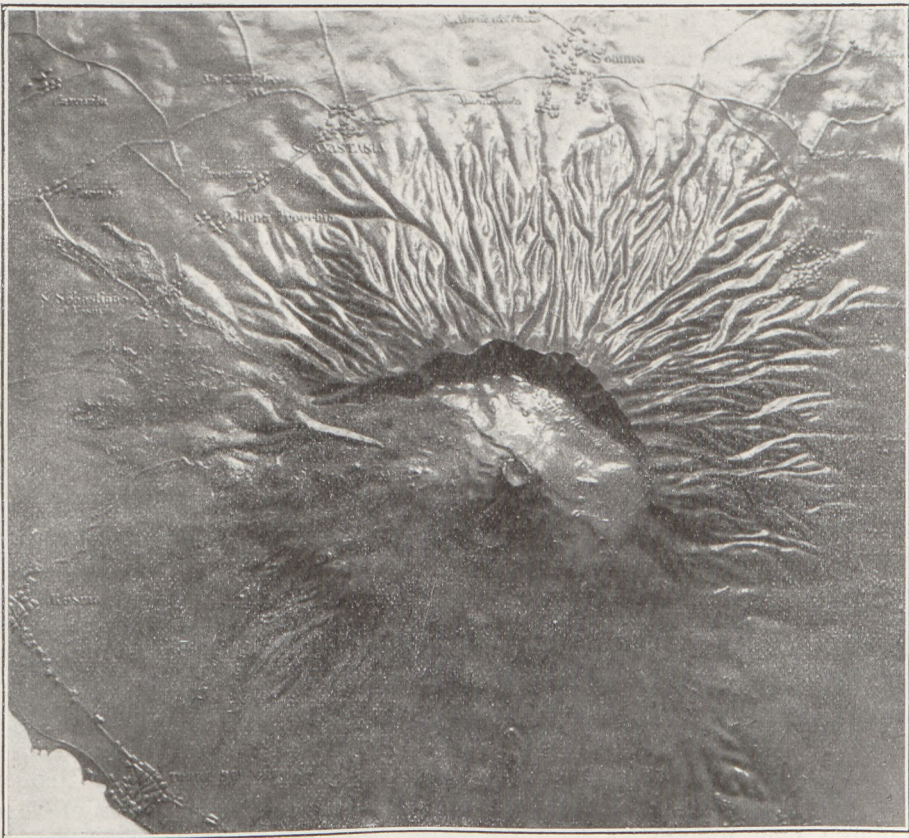
Fig. 86 Vesuv mit Somma aus der Vogelschau, nach einem Modell von A. Aureli
