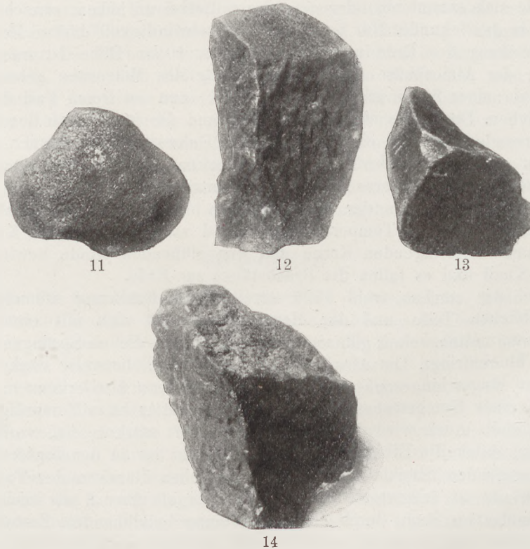
Fig. 11—14 Bruchstücke des Meteorsteinfalles von Mées
