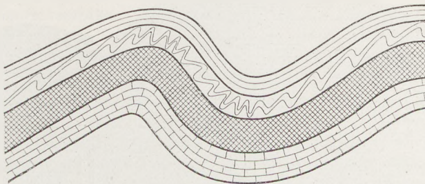
Fig. 169 Unharmonische Faltung
