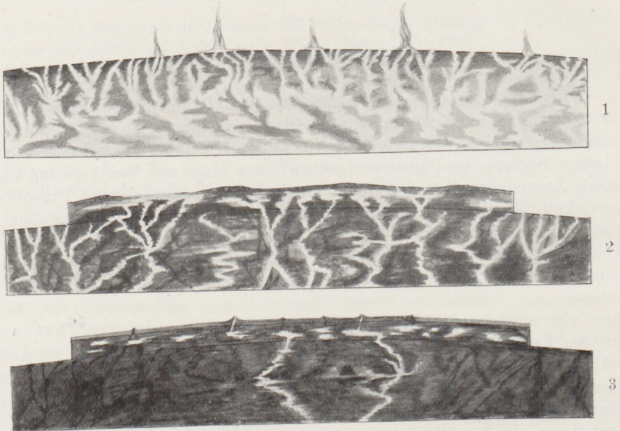
Fig. 1—3 Die Bildung der festen Erdrinde (nach A. Stübel)
