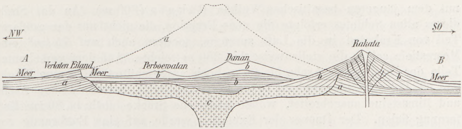
Fig. 79 Durchschnitt durch Krakatau vor dem Ausbruche 1883 nach A, B in Fig. 78 (nach R. D. M. Verbeek). a Reste des ursprünglichen Kegels und dessen Ergänzung, b jüngere Vulkankegel, c Lava in der alten Caldera
