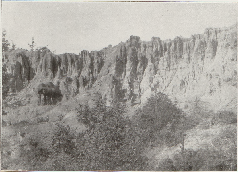
Fig. 250 Erdpyramiden bei Daničići, Bosnien (phot. F. Wähner)
