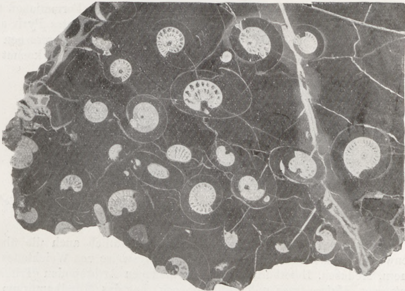
Fig. 454 Ammonitenkalkstein. Die Luftkammern der Gehäuse sind zum Teil mit weißem Kalkspat erfüllt, zum Teil Hohldrüsen.
