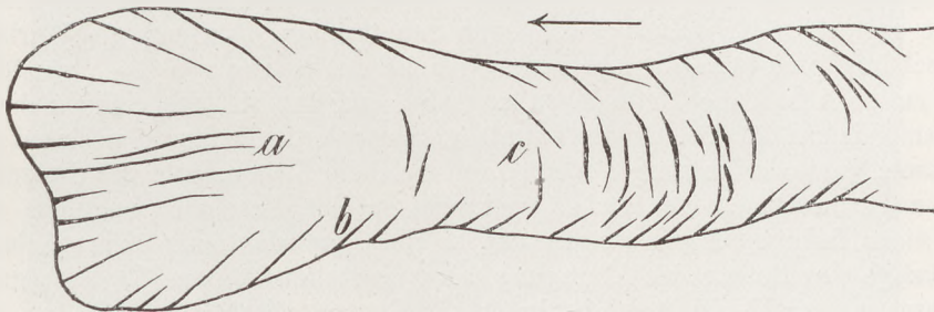
Fig. 323 a Längsspalten, b Randspalten, c Querspalten im Gletscher
