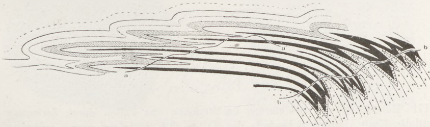
Fig. 168 Überfaltungsdecken, die in den Profilen a—a' und b—b' abgetragen sind, sodaß unter b—b' die Wurzelregion erhalten ist (nach M. Bertrand und E. Ritter).
