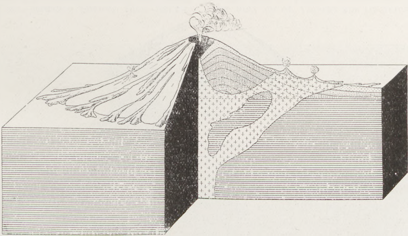
Fig. 50 Modell des Vesuv. Zeigt die Schichtung des Kegels, die radialen Gänge, den Krater, parasitäre Kegel und Lavaströme auf den Flanken.
