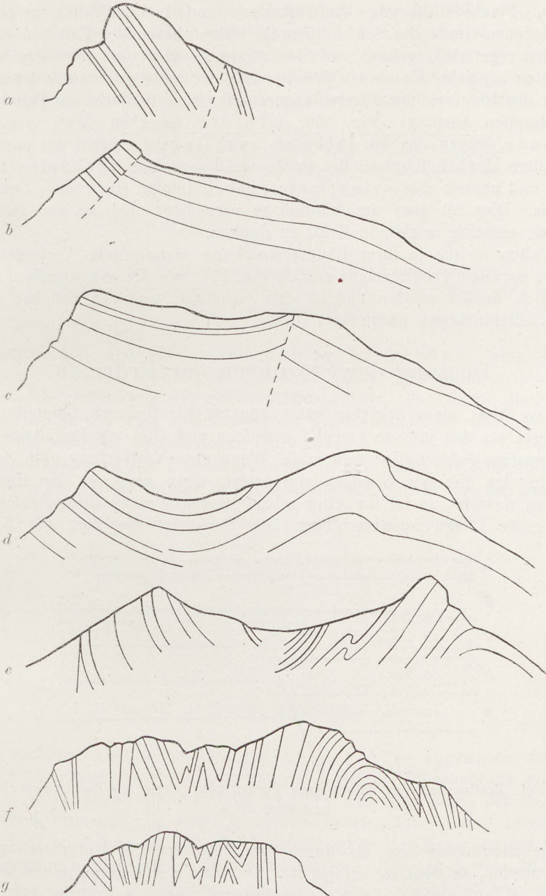
Fig. 157 Veränderung eines Faltenzuges in der Längerstreckung. Während bei a gleichsinniges Fallen, nur durch eine Verwerfung unterbrochen, besteht, stellt sich allmählich eine flache Falte ein, die enger zusammengepreßt wird (nach A. Buxtorf).
