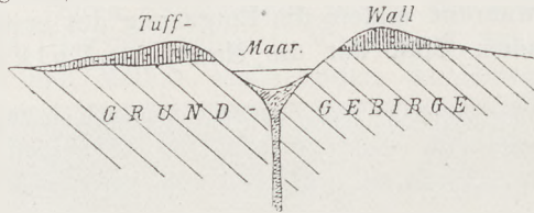
Fig. 67 Idealer Durchschnitt durch ein Eifler Maar (nach F. von Wolf)
