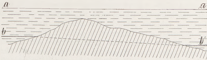
Fig. 283 Entstehung eines epigenetischen Tales. Der Fluß ist zuerst im Niveau a a' geflossen und durchschneidet bei seiner Tieferlegung im Niveau b b' eine begraben gewesene Erhebung des Untergrundes.
