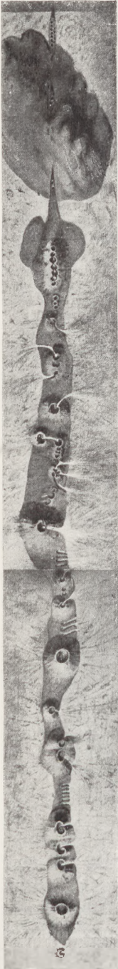
Fig. 109 Lakispalte mit aufgesetzten Vulkankegeln (nach A. Helland)
