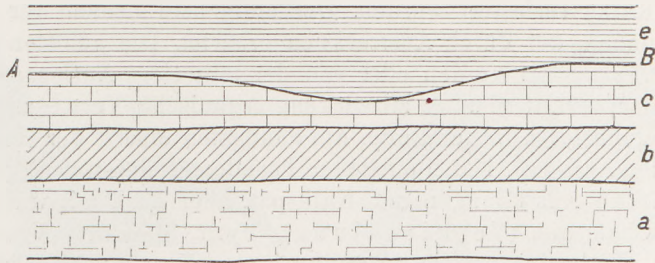
Fig. 405 Erosionsdiskordanz; nach Ablagerung der Schichten a—d (vgl. Fig. 160) erfolgte Erosion und Ablagerung von e auf der Abtragungsfäche A—B .
