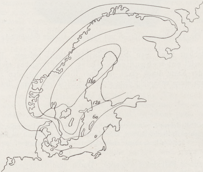
Fig. 119 Die nacheiszeitlichen Hebungen in Skandinavien. Die Kurven verbinden die um den gleichen Betrag (in Metern ausgedrückt) gehobenen Punkte (Isoanabasen) (nach G. de Geer).
