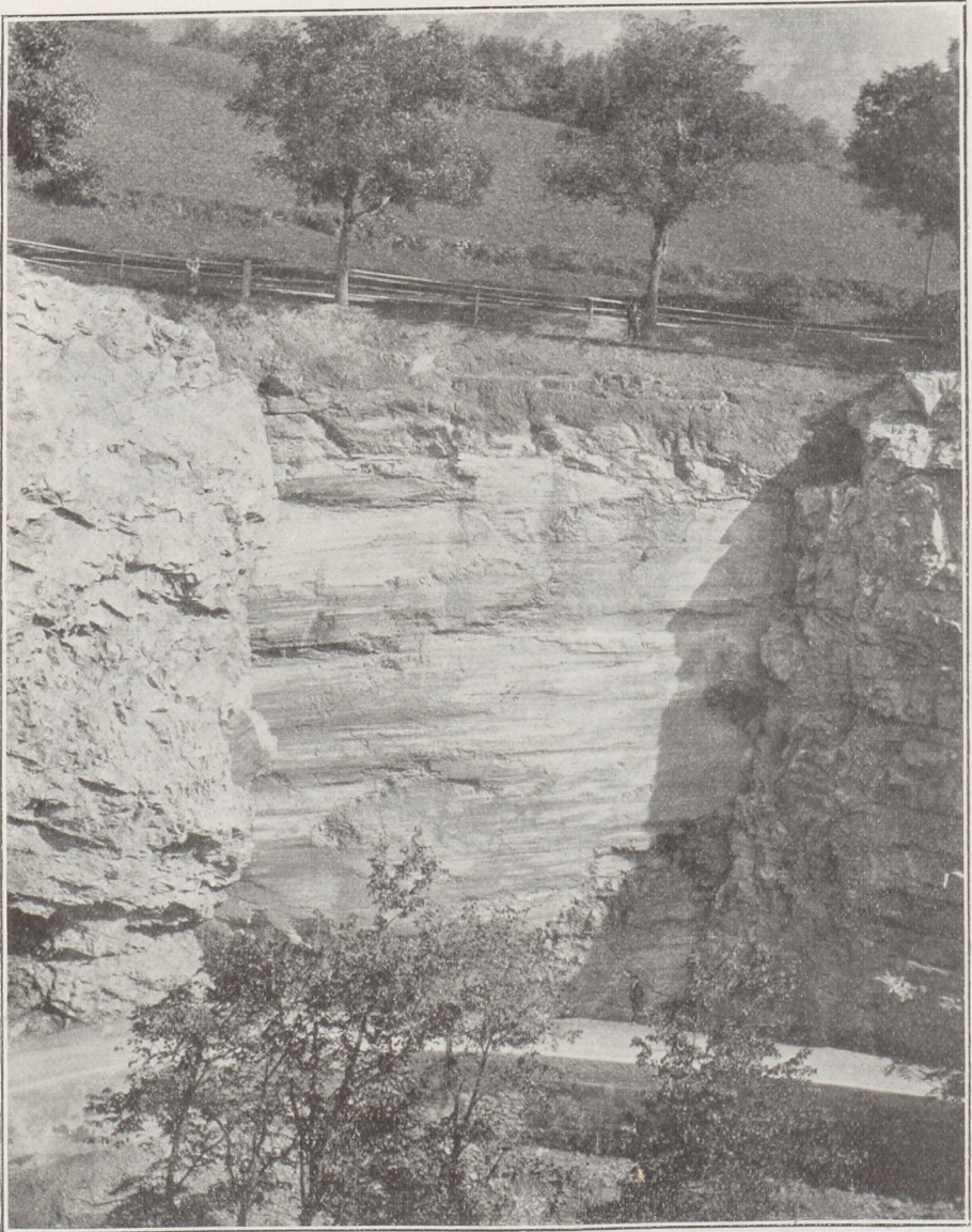
Fig. 143 Blattverschiebung mit Harnisch. Gamperleloch an der Kapfstraße bei Feldkirch in Vorarlberg (nach einer Aufnahme von J. Niggli, Feldkirch)
