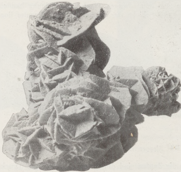
Fig. 416 Gipsdruse aus dem Wüstenboden vom Schott el Mreir, Algier
