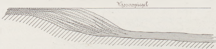
Fig. 400 Längsschnitt durch ein Delta
