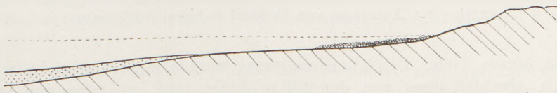
Fig. 313 Endgestalt des Strandgebietes bei fortschreitender mariner und subaërischer Abtragung
