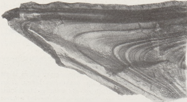
Fig. 170 Bruchlose Faltung in Tonschiefer
