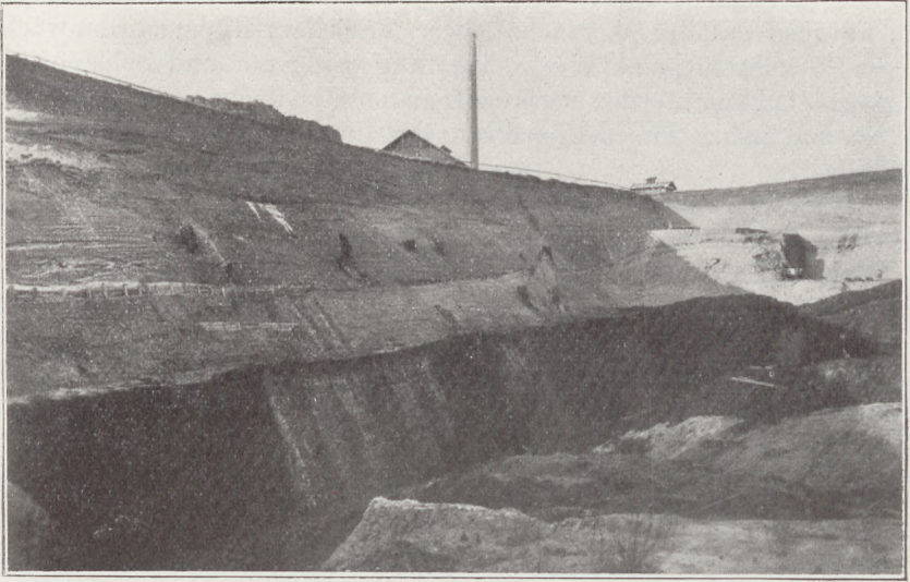
Fig. 385 Allochthones Braunkohlenflöz bei Zillingsdorf, Niederösterreich. Im Hangenden Sande mit Kreuzschichtung und aufrechten Baumstämmen (phot. Langer & Co., F. Hrdlička, G. m. b. H., Wien)
