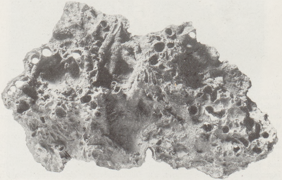
Fig. 379 Kalktuff mit Stengelröhren
