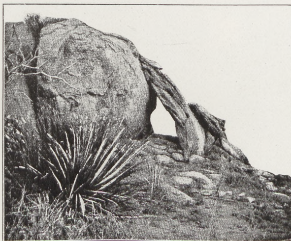
Fig. 215 Abschuppung eines Granitblockes (nach G. von dem Borne aus J. Walther)
