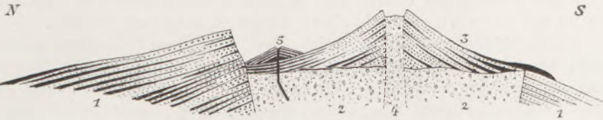
Fig. 85 Profil durch Vesuv und Somma (nach F. Löwl). 1 Reste des alten Somma-vulkanes mit Lavaergüssen, 2 der mit Brockentuff gefüllte Schlot, 3 Vesuvkegel mit Lavaergüssen, 4 der heutige Schlot, 5 parasitärer Lavakegel im Atrio
