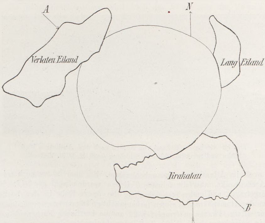
Fig. 80 Karte von Krakatau nach dem Ausbruche 1883 (nach R. D. M. Verbeek)
