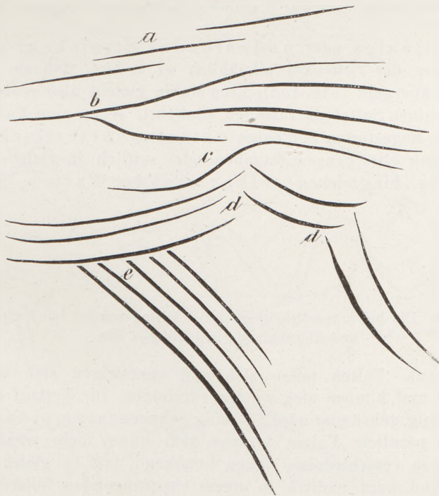
Fig. 154 Faltenleitlinien. a vikariierende Falten, b Virgation, c sigmoidale Beugung, d , d Scharung, e ein Faltensystem wird durch ein jüngeres quer verlaufendes gekreuzt und taucht darunter.
