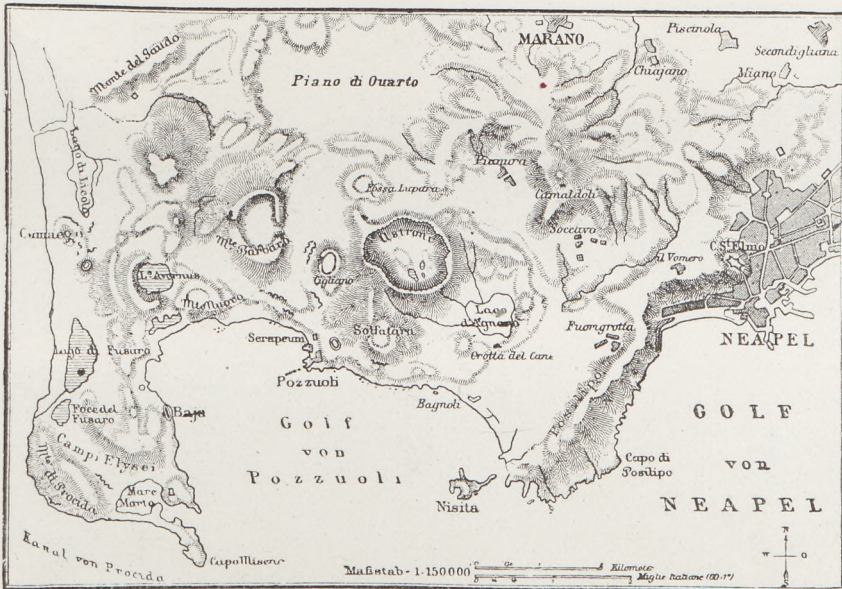
Fig. 91 Karte der Phlegräischen Felder (nach M. Neumayr)
