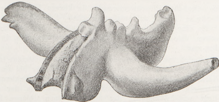
Fig. 464 Kerunia (nach E. Fraas)
