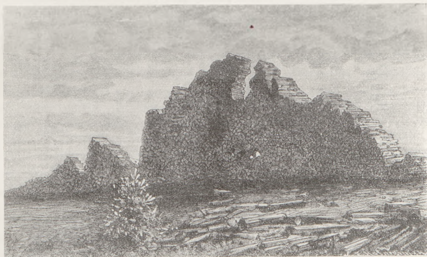
Fig. 116 Die Teufelsmauer in Nordböhmen (nach Wurm aus F. Löwl)
