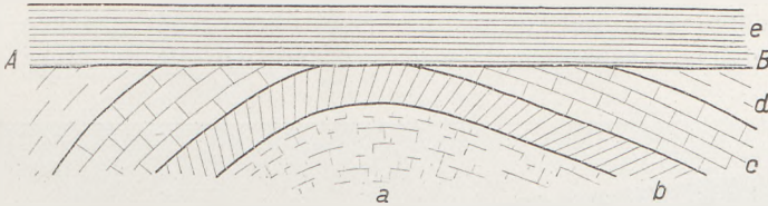
Fig. 159 Bestimmung des Alters einer Faltung, jünger als das Schichtglied d und älter als e . A—B ist eine Abtragungsfäche, auf der e diskordant aufliegt. Die Schichten a—d liegen konkordant.
