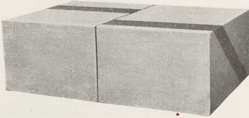
Fig. 130 Querverwerfung nach Abtragung des Hangendflügels
