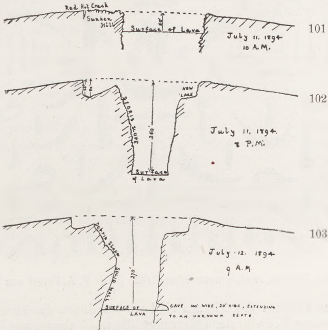
Fig. 101—103 Querschnitte durch den Halemauau, die Schwankungen der Lava und Nachbrüche zeigend. (nach W. T. Brigham)
