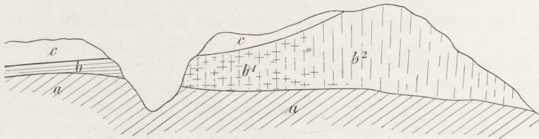
Fig. 422 Indirekter Beweis der Altersgleichheit von Schichten. b geht allmählich in das petrographisch verschiedene b 1 und b 2 über und kann nur durch die Lagerung zwischen a und c wieder erkannt werden.
