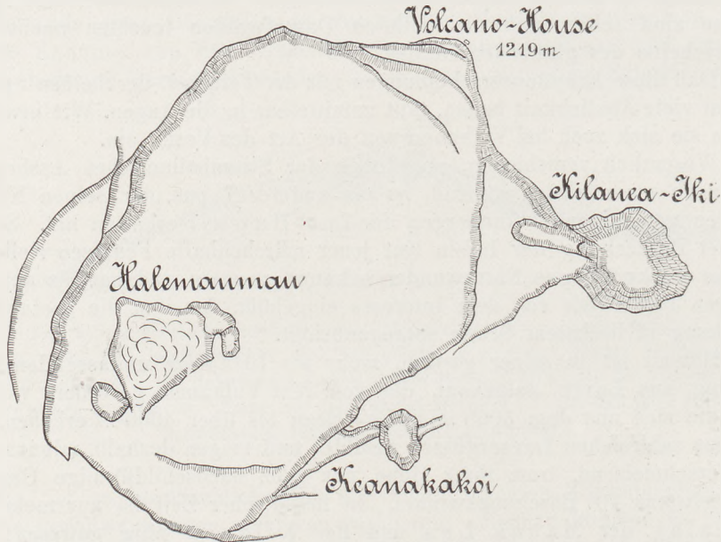
Fig. 98 Karte des Kilauea-Kraters (nach J. D. Dana). Zeigt den großen Krater mit dem Halemauau im Innern und die zwei kleineren im Osten.
