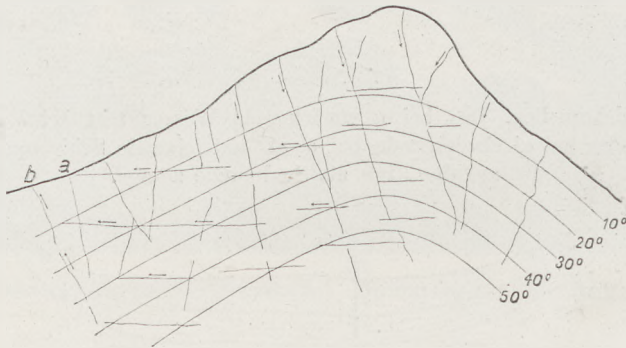
Fig. 303 Das an der Oberfläche in Klüfte einsickernde Wasser nimmt die Temperatur der Geoisothermen an und tritt bei a als absteigende, bei b als aufsteigende Quelle (bzw. Therme) zutage.
