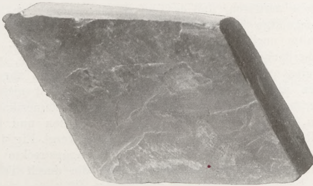
Fig. 176 Durch Diaklasen begrenzte Schieferplatte
