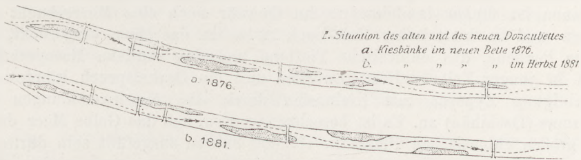
Fig. 261 Wandern der Sandbänke im regulierten Donaubette bei Wien (nach J. Lorenz von Liburnau, aus R. Hörnes)
