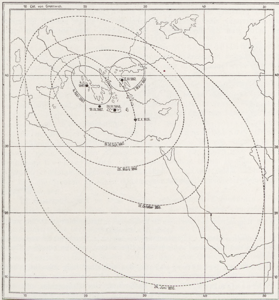
Fig. 188 Verbreitungsgebiete der großen orientalischen Erdbeben (nach J. Schmidt aus R. Hörnes). Für das Erdbeben 1870 ist das Epizentrum nicht angedeutet.
