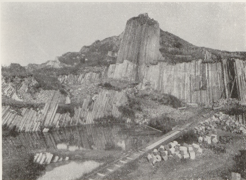
Fig. 58 Herrnhäuser Stein bei Steinschönau, Böhmen. Säulenförmig abgesonderter Basalt (nach einer Aufnahme von H. A. Eckert)
