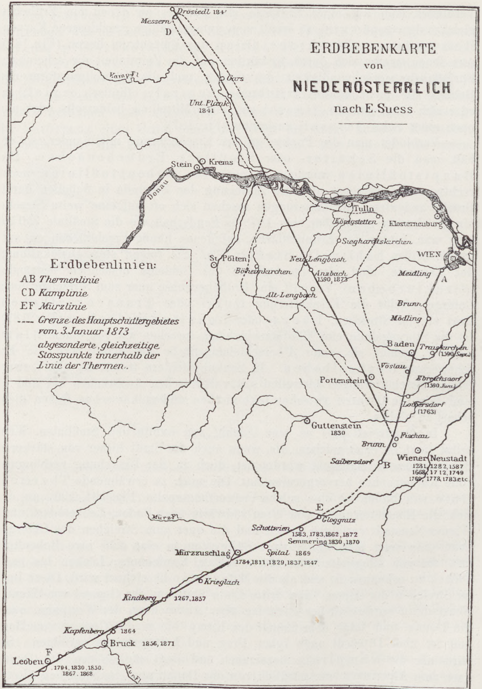
Fig. 190 Erdbebenkarte von Niederösterreich nach E. Suess (aus R. Hörnes)
