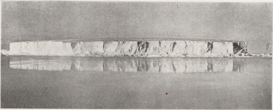
Fig. 334 Tafelförmiger Eisberg, Antarktis (nach E. Philippi)
