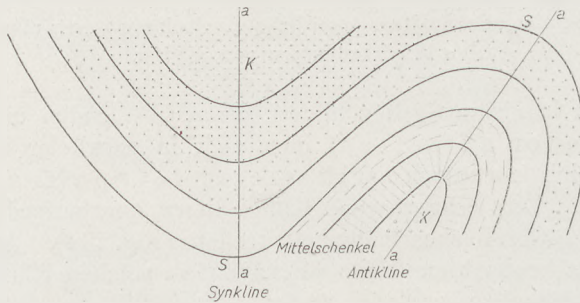
Fig. 147 Mulde und Sattel. a—a Achsen, S Scheitel, K Kerne
