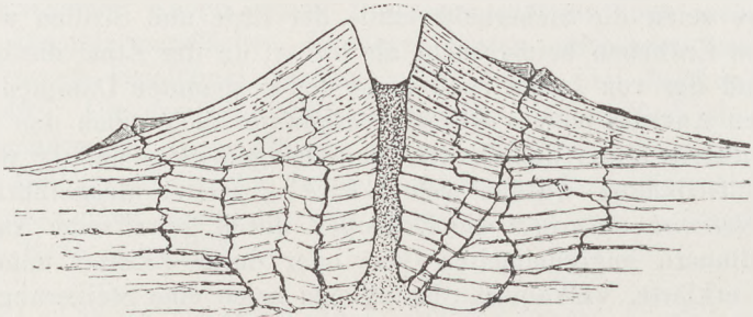
Fig. 41 Idealquerschnitt durch einen durch wiederholte Ausbrüche entstandenen Vulkan (nach P. Scrope)
