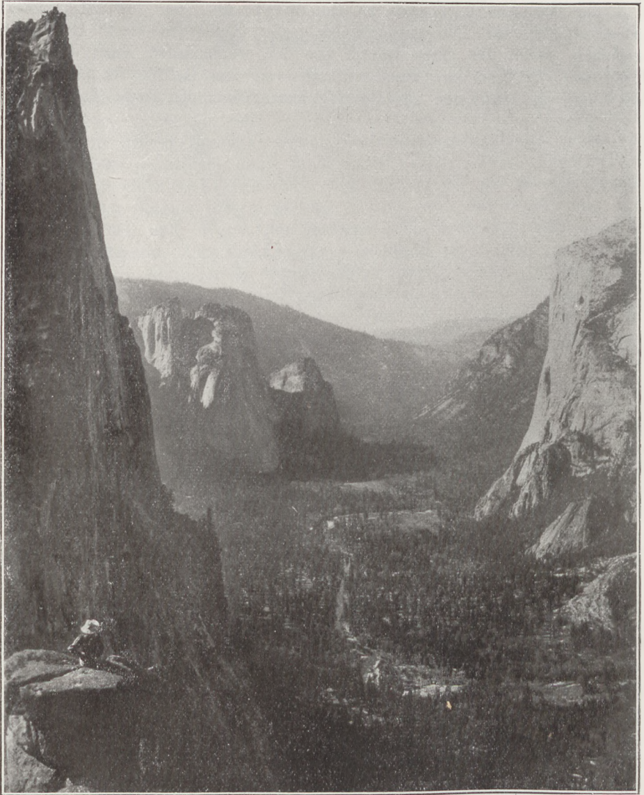
Fig. 337 Yosemitetal in Kalifornien (U-Tal) (nach einer käuflichen Photographie)
