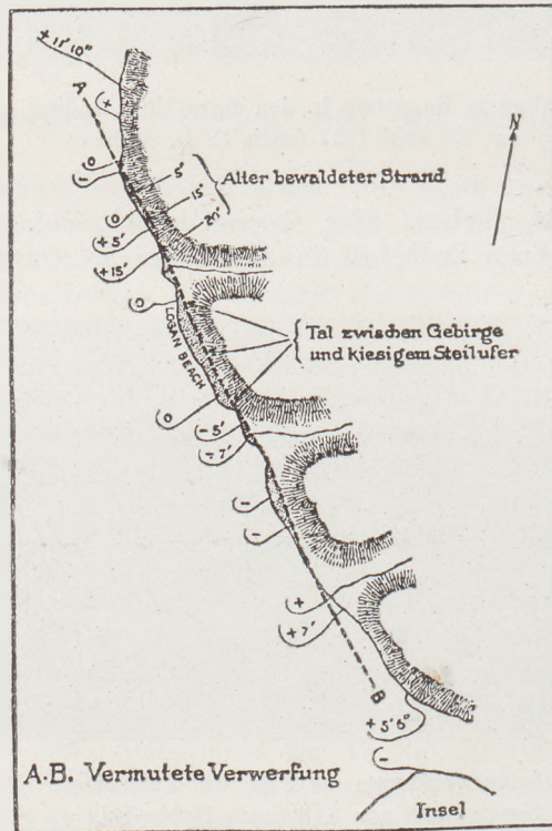
Fig. 195 Positive und negative Verschiebungen der Strandlinie an der Yakutat Bay (nach Tarr und Martin aus Hobbs-Ruska)
