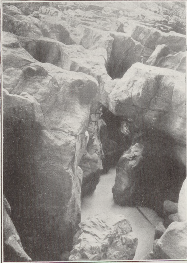
Fig. 263 Erosion der Sarca bei Ponte Balantino, Südtirol (nach einer Aufnahme von G. B. Unterveger, Trient)
