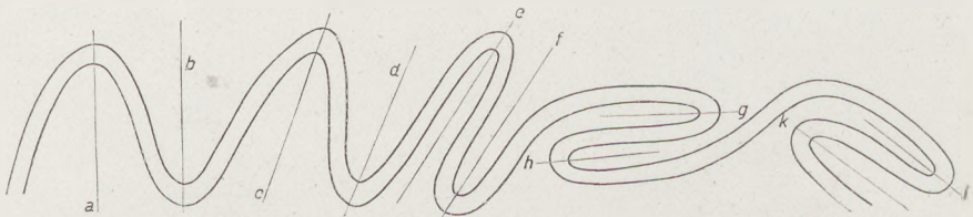
Fig. 148 Lage der Falten. a aufrechter Sattel, b aufrechte Mulde, c schiefer Sattel, d schiefe Mulde, e überkippter Sattel, f überkippte Mulde, g, h liegende Falte, i überstürzter Sattel (falsche Mulde), k überstürzte Mulde (falscher Sattel)
