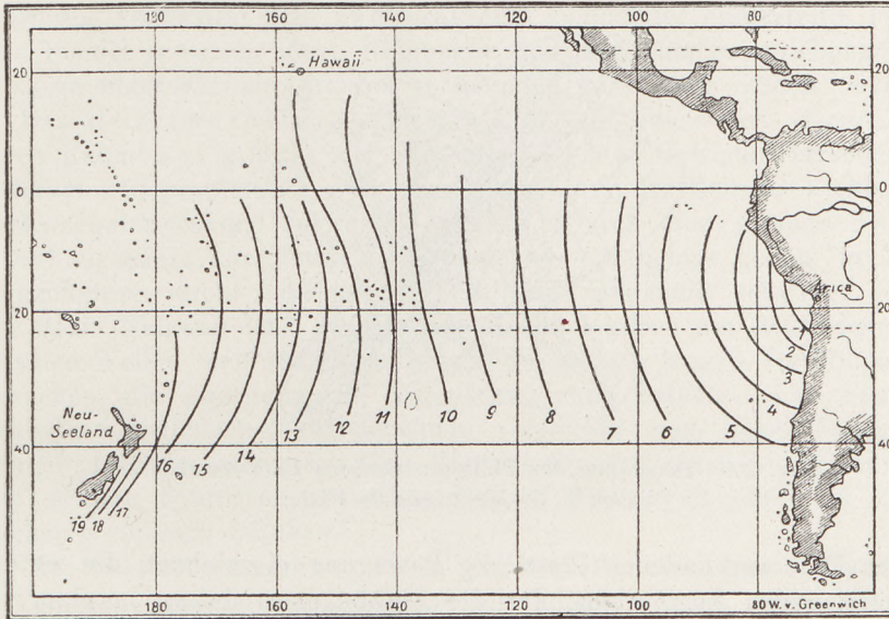
Fig. 208 Verbreitung der Erdbebenflutwelle vom 13. August 1868 im Pazifischen Ozean (nach F. v. Hochstetter aus R. Hörnes). Die Zahlen geben die Lage der Welle in Stunden nach dem Beben von Arica an.
