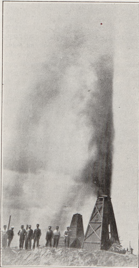
Fig. 389 Ölspringer in Balachany, Transkaskasien (nach einer käuflichen Photographie)
