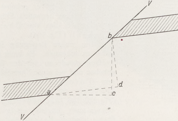
Fig. 123 Verwerfung einer Schicht durch eine Kluft V-V . a-b ist die flache, b-c die seigere, b-d die wirkliche Sprunghöhe.
