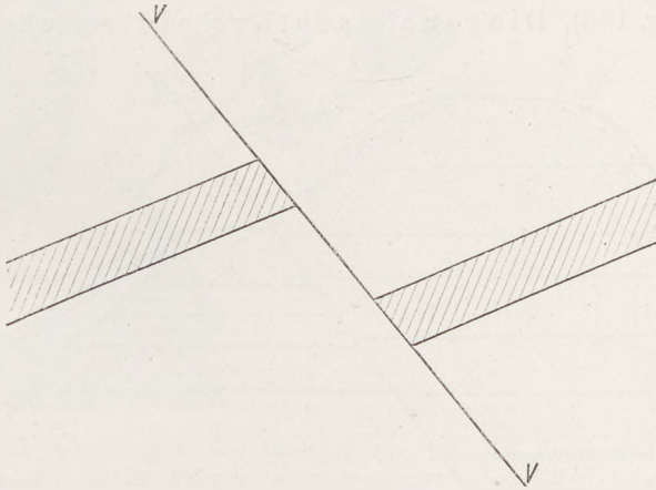
Fig. 131 Widersinnig fallende Verwerfung V-V . Ist der über der Kluft liegende (rechte) Flügel nach oben verschoben, so entsteht eine widersinnige Überschiebung.
