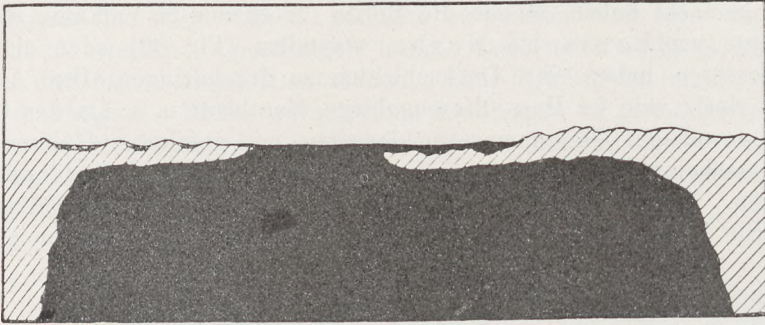
Fig. 31 Arealeruption (nach F. von Wolff). Das Magma (schwarz) durchbricht die Erdkrinde (schrattiert) und ergießt sich über die Oberfläche.
