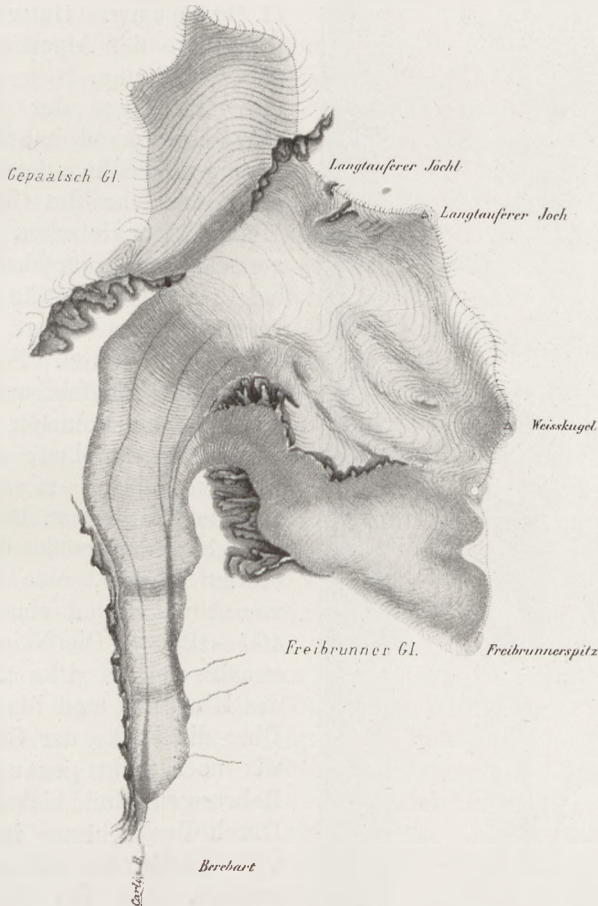
Fig. 320 Nähr- und Zehrgebiet des Langtaufere Gletschers, Tirol (nach K. v. Sonklar)
