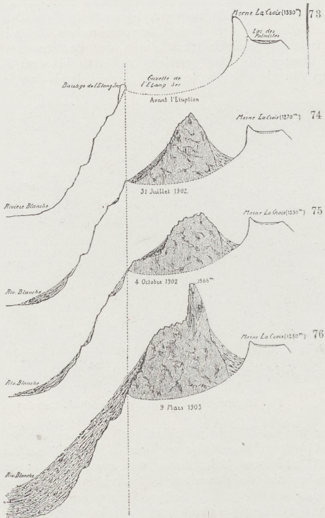
Fig. 73—76 Entwicklung des Domes und der Nadel der Montagne Pelée (nach A. Lacroix)
