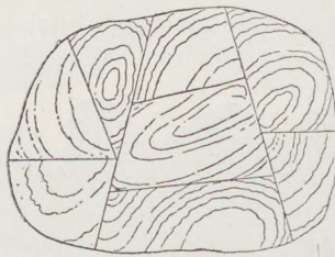
Fig. 233 Farbenringe in einem von Spalten durchschnittenen Kalkblocke (nach J. Walther)
