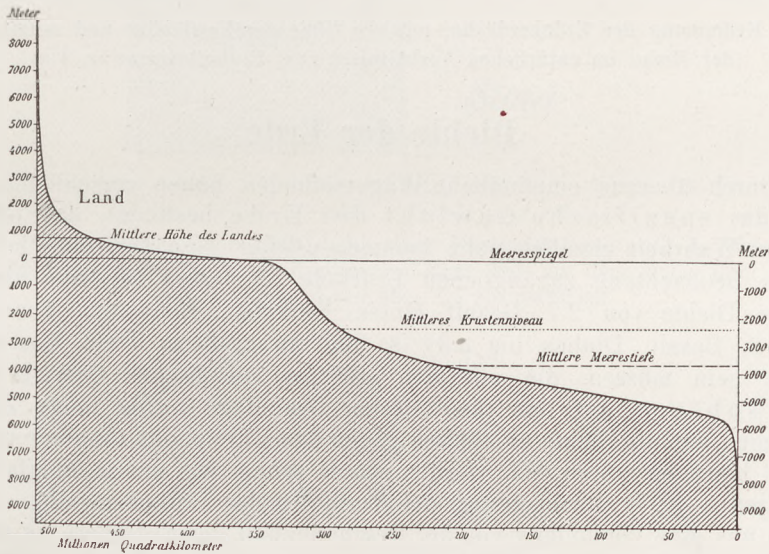
Fig. 4 Hypsographische Kurve der Erdoberfläche (nach O. Krümmel). Verhältnis der Höhe, Oberfläche und Masse des Festlandes zur Tiefe, Oberfläche und Masse des Weltmeeres
