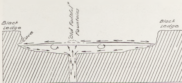
Fig. 104 Konvektionsströmungen im Halemauau (nach R. A. Daly)
