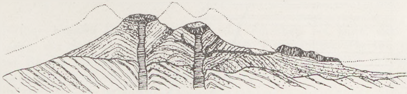
Fig. 113 Profil durch die vulkanischen Necks des Largo Law, Fife (nach A. Geikie)
