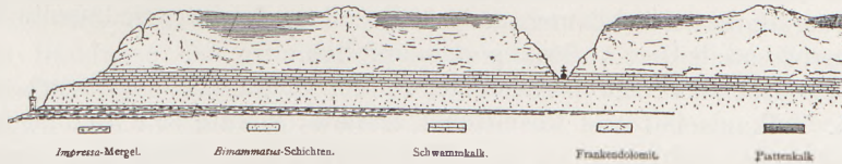
Fig. 395 Profil durch die jurassischen Kalkriffe von Pappenheim bis Eichstädt, Altmühl-gegend, Bayern. Verzahnung der in Lagunen abgelagerten Plattenkalke mit den Riffkalken (nach J. Walther)
