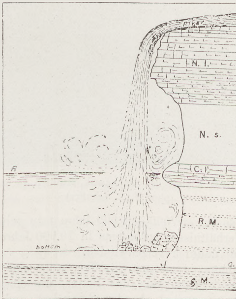
Fig. 265 Profil des Niagarafalles (nach J. W. W. Spencer). Die leicht zerstörbaren schiefrigen Schichten R. M. und N. s. werden ausgewaschen und der feste Kalkstein N. l. bricht nach.
