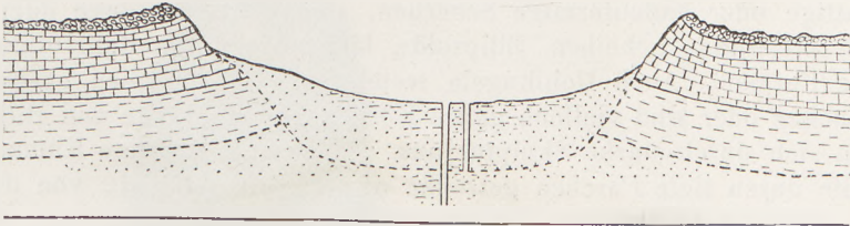
Fig. 19 Profil durch den Meteor Crater (nach N. H. Darton)
