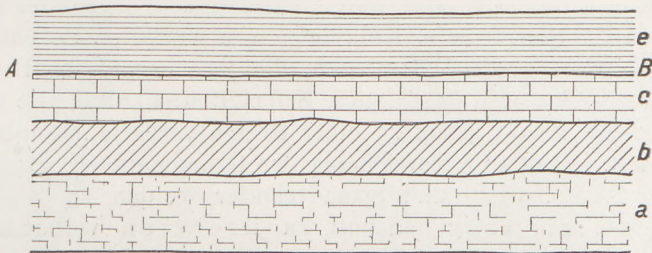
Fig. 406 Maskierte Diskordanz; die Abtragungsfäche A—B entspricht einer Schichtfläche und wird Auflagerungsfläche.
