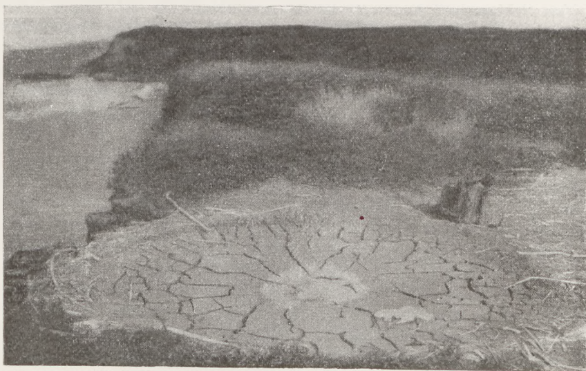
Fig. 387 Schlammquelle auf einem Mudlump (nach E. W. Shaw)
