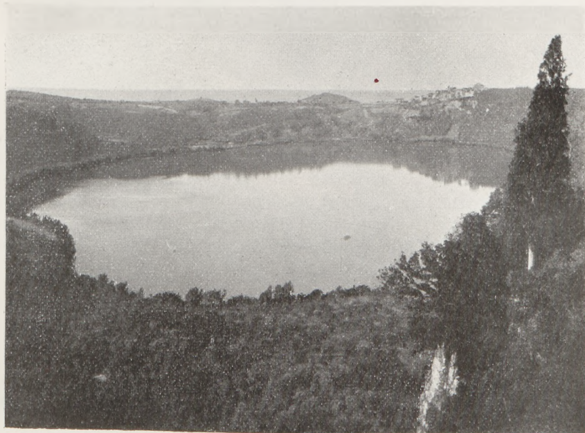
Fig. 66 Lago di Nemi, ein Maar im Albanergebirge (nach einer Aufnahme von G. Sommer, Neapel)
