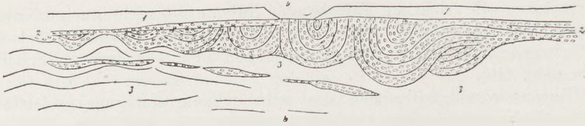
Fig. 245 Durch Rutschung entstandene Störungen im Schotter des Laaerberges in Wien (nach Th. Fuchs). 1 Löss, 2 Laaerbergsschotter, 3 Congerientegel, b-b 8 m.
