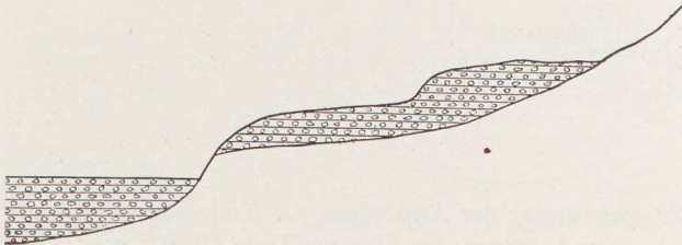
Fig. 275 Zwei ältere Auftragsterrassen, darunter Einschneiden des Flusses bis auf den Untergrund und Aufschüttung eines jüngeren Schotterbettes
