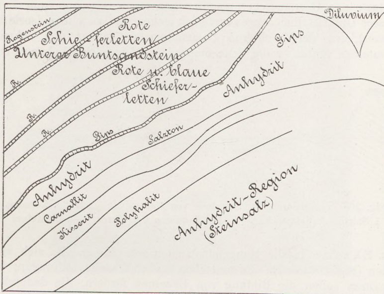
Fig. 365 Profil durch das Staßfurt-Leopoldshaller Salzlager (nach F. A. Fürer)
