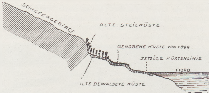
Fig. 194 Drei übereinander liegende Strandterrassen am Russel-Fjord, um 1·3 und 3 m gehoben (nach Tarr und Martin aus Hobbs-Ruska).
