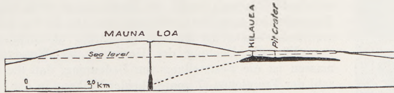
Fig. 107 Vermutete Lakkolithen als Quelle der vulkanischen Tätigkeit des Kilauea und Mauna Loa (nach R. A. Daly)
