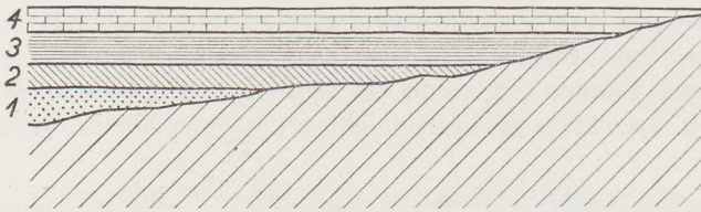
Fig. 423 Profil einer Schichtfolge bei Transgression
