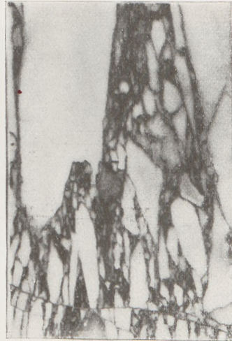
Fig. 174 Gestreckte Breccie
