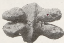
Fig. 477 Walnußkern, als Reliefsteinkern erhalten
