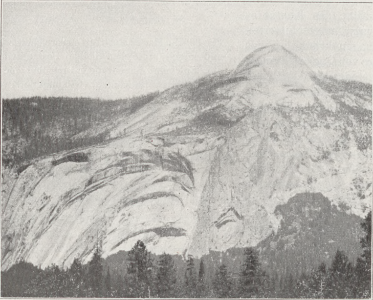
Fig. 39 Kugelschalenförmige Absonderung des Granits im Yosemite-tale, Kalifornien (phot. F. X. Schaffner)
