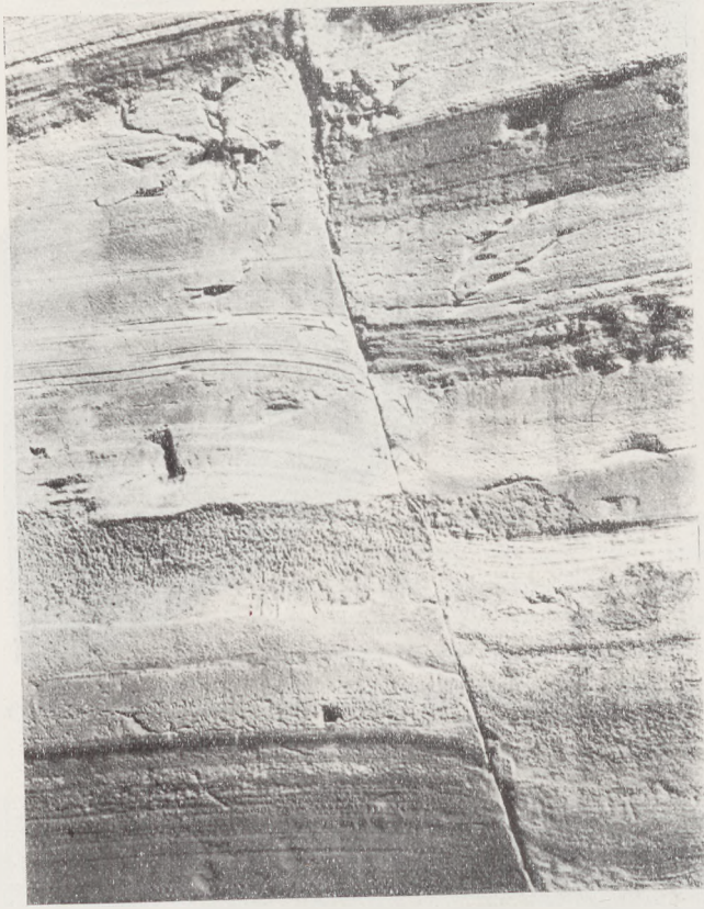
Fig. 128 Verwerfung und Schleppung am Kanal von Korinth (Aufnahme von F. X. Schaffer)
