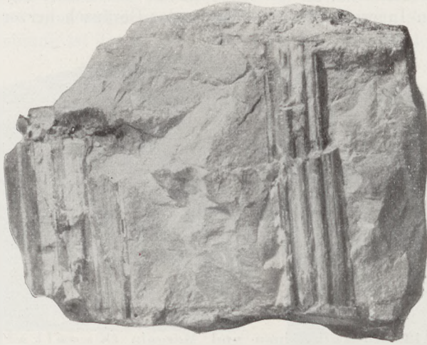
Fig. 415 Stylolithen
