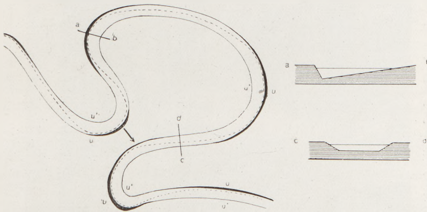
Fig. 271 Flußschlinge, die in der Richtung des Pfeiles durchrissen wird. u Prallufer, u' Anwachsuf, Stromstrich gestrichelt. Profil a—b in einer Krümmung, c—d in geradem Stromlaufe
