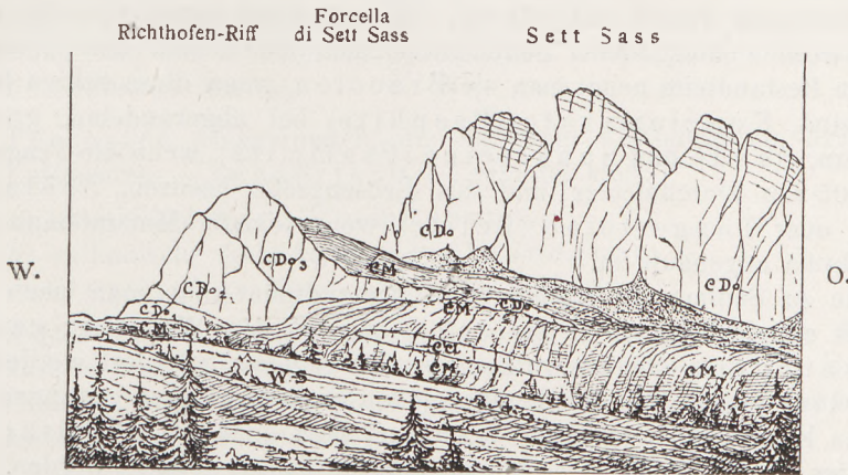
Fig. 394 Riffverzahnung am Sett Sass, Südtirol. Auskeilen eines Riffes in mergeligen Schichten (nach E. von Mojsisovics)
