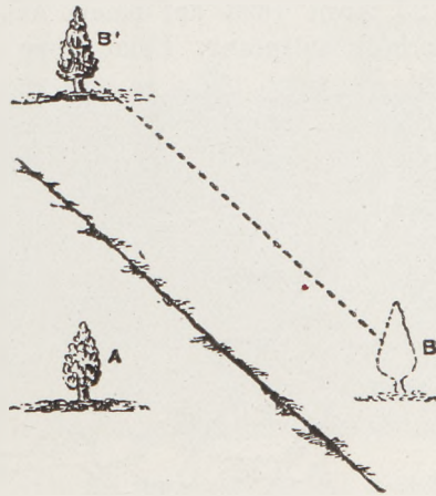
Fig. 196 Horizontale Verschiebung an der Neo-Tal-Verwerfung bei Idbara (nach Kotô aus Hobbs-Ruska)
