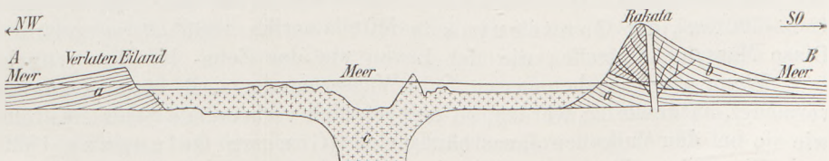
Fig. 81 Durchschnitt durch Krakatau nach dem Ausbruche von 1883 nach A, B in Fig. 80 (nach R. D. M. Verbeek). Die alte Caldera ist wieder hergestellt.
