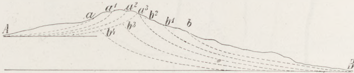
Fig. 269 Rückverlegung der Wasserscheide von b nach b^4 durch die stärkere Erosion des Flusses b-B
