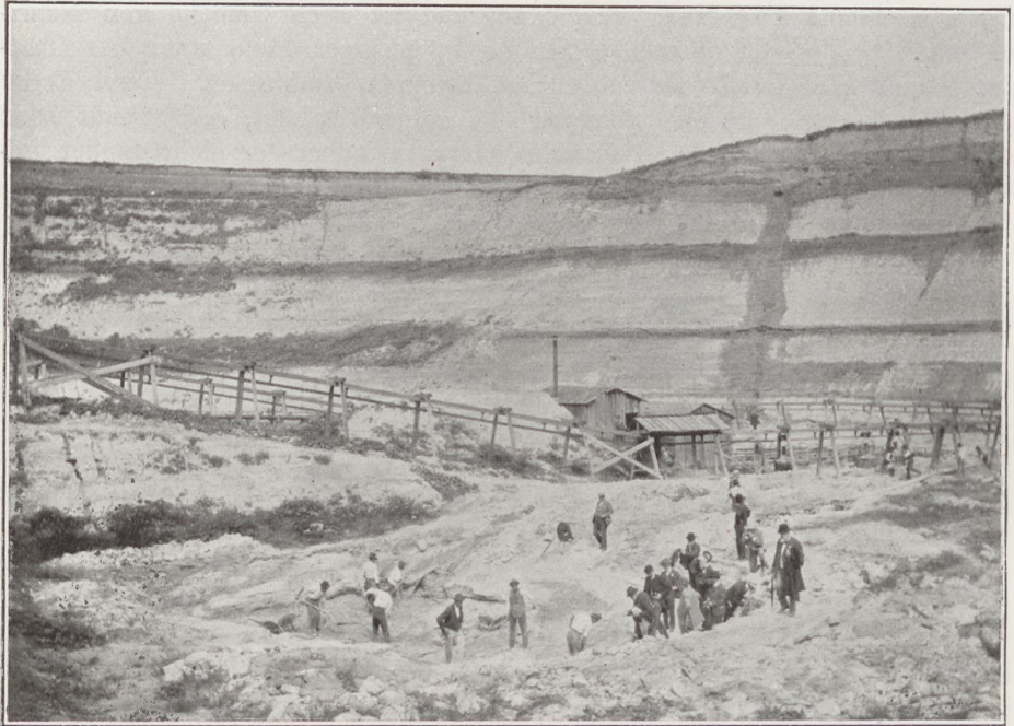
Fig. 289 Wasserführende Horizonte (dunkel) an der Grenze zweier verschieden durchlässiger Schichten im Congerientegel bei Wien (phot. F. X. Schaffer)
