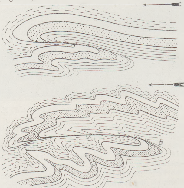
Fig. 151, 152 Faltenüberschiebung durch Auswalzung des Mittelschenkels (längs A—B) der in der Richtung des Pfeiles bewegten liegenden Falte
