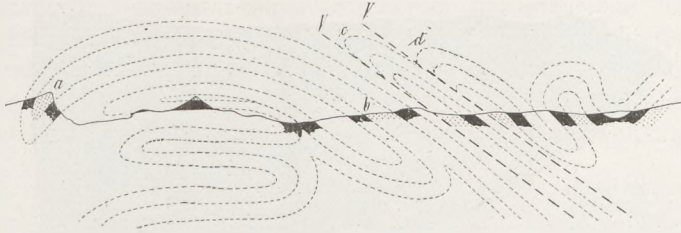
Fig. 167 Abgetragenes Faltenhochgebirge. Die ausgezogenen Linien zeigen an, wieweit eine Beobachtung des Baues möglich ist. Die punktierten Linien geben die Rekonstruktion der Falten. a Stirn einer Überfaltung; die weiter rechts sichtbare horizontale Lagerung ist keine ursprüngliche, sondern eine liegende Falte. Bei b folgen inverse und normale Lagerung aufeinander. Durch die Überschiebungen V, V' entsteht eine Wiederholung der normalen Schichtfolge in c und d (Schuppenstruktur).
