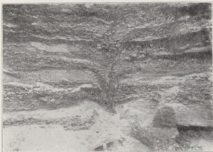
Fig. 207 Erdbebenspalte in einer Kiesgrube bei Heidelberg, junges Diluvium (Aufnahme von W. Spitz aus Hobbs-Ruska)
