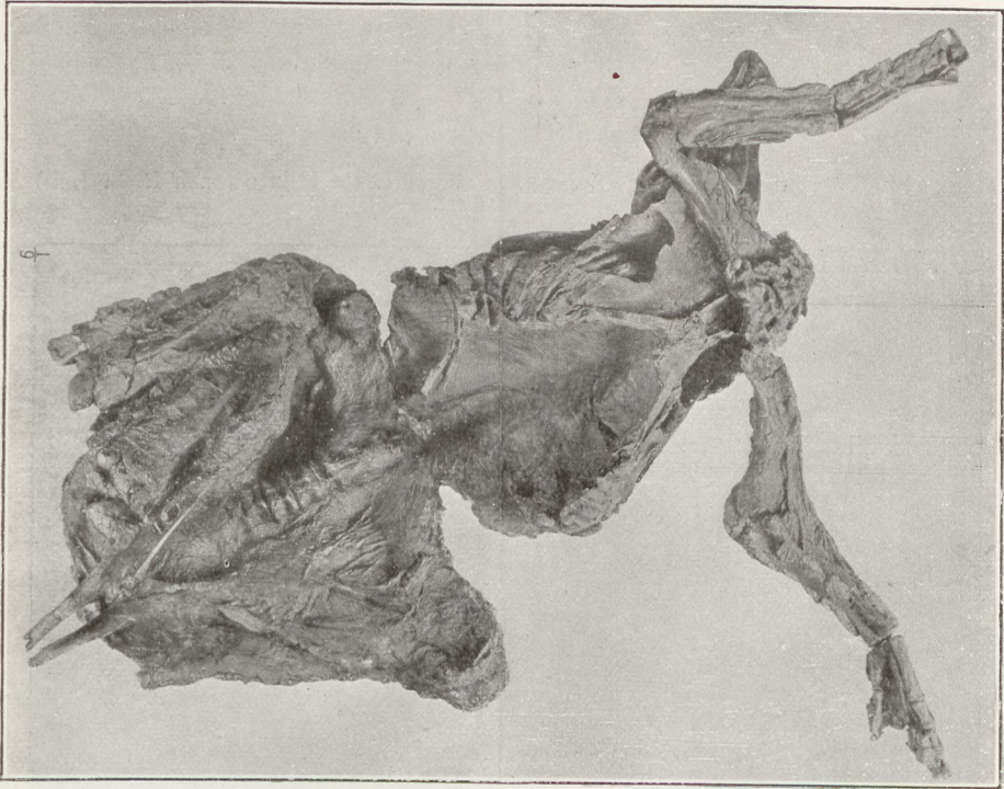
Fig. 439 Fossile Mumie von Trachodon , eines Dinosauriers aus der oberen Kreideformation von Wyoming, Nordamerika (nach H. F. Osborn)
