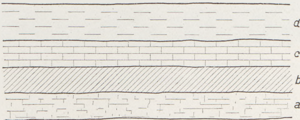
Fig. 160 Ungestörte, konkordante Lagerung
