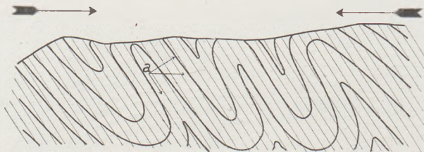
Fig. 171 Entstehung von Schieferung im Streichen von Falten durch Zerlegung der tangentialen Kraft. In den Schenkeln der Falten fällt Schieferung und ursprüngliche Schichtung zusammen, in den Scheiteln kann Griffelstruktur entstehen.
