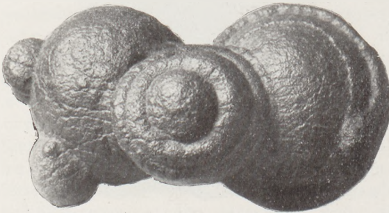
Fig. 412 Brauneisensteinkonkretion
