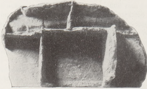
Fig. 410 Spaltausfüllungen von Quarz, durch Verwitterung herausgearbeitet.
