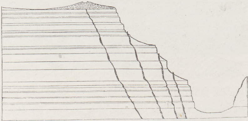
Fig. 115 Vulkanische Stiele am Grand Kanyon des Colorado N. A. (nach C. E. Dutton)
