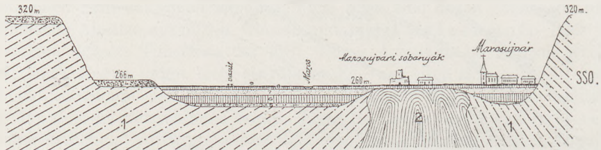
Fig. 366 Profil durch den Salzstock von Marosujvár (nach Th. Kormos) 1 Salzton, 2 Salzstock, 3—4 alte Terrassen der Maros, 5—9 Alluvium
