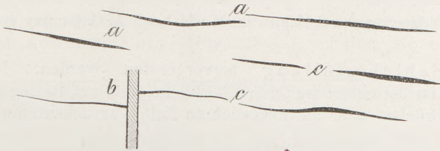
Fig. 144 a vikarierende Spalten, b seitliche Auslenkung durch eine ältere Klüft, c Wiederaufsetzen von Spalten
