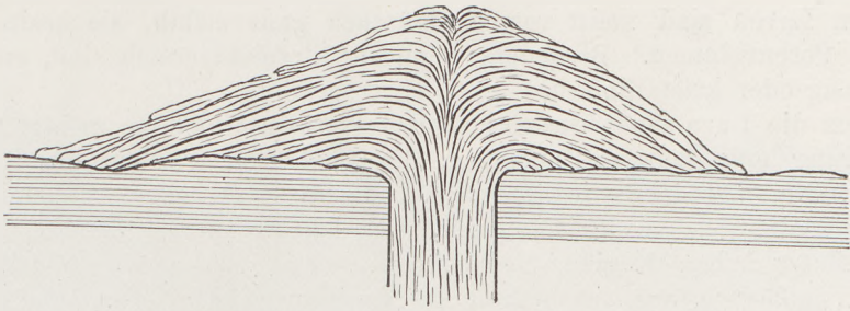
Fig. 54 Quellkuppe, durch Überfließen entstanden
