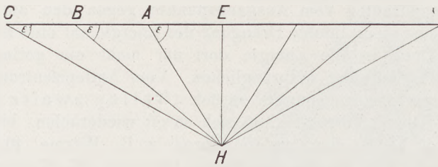
Fig. 186 Emergenzwinkel ( \epsilon ), H Hypozentrum, E Epizentrum, A , B , C Punkte der Erdoberfläche
