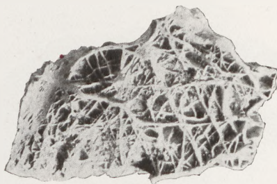
Fig. 408 Zellendolomit
