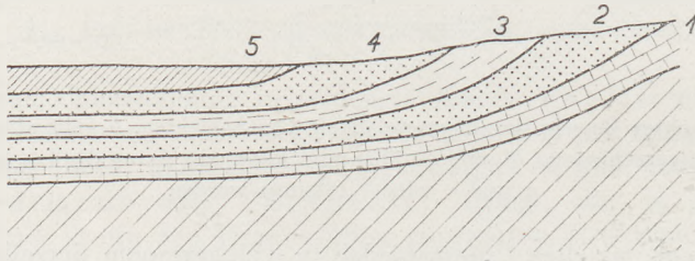
Fig. 424 Profil einer Schichtfolge bei Regression
