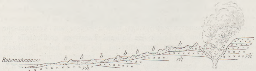
Fig. 373 Querschnitt durch die Sinterterrassen des Rotomahanasees (nach F. v. Hochstetter) a Hauptbecken, b die Becken der Terrassen, c Sinterbildungen, rh Rhyolith
