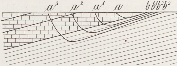
Fig. 280 Seitliche Verlegung eines Flußlaufes im Schichtfallen infolge größerer Widerstandsfähigkeit der Liegendschichten. a-b bis a^3-b^3 zeitlich aufeinander folgende Profile des Tales
