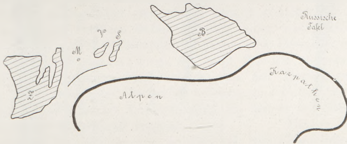
Fig. 178 Leitlinie der Alpen und Karpathen, bestimmt durch die alten Massen des französischen Zentralplateaus (Z), der Masse von Dôle (M), der Vogesen (V), des Schwarzwaldes (S), der böhmischen Masse (B) und der russischen Platte.
