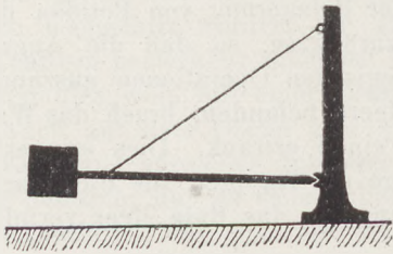
Fig. 210 Prinzip des Horizontalpendels (nach F. de Montessus de Ballore)
