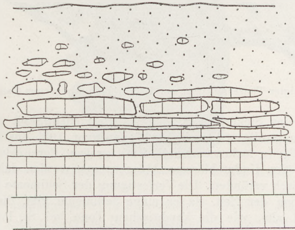
Fig. 418 bergang von losem Sediment in festes Gestein durch Verkonkretionierung
