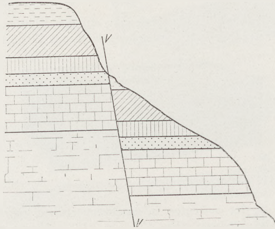
Fig. 132 Wiederholung von Schichtgliedern (1—4 von oben) im Profile durch eine Verwerfung V—V
