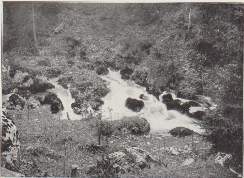
Fig. 300 Schreierquelle bei Hinterwildalpen (Aufnahme von Th. Mark, Scheibbs)
