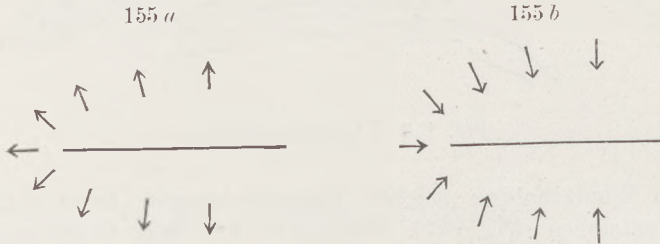
Fig. 155 Periklinales Streichen: a an einem Sattelenende, b an einem Muldenende
