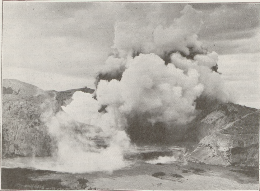
Fig. 308 Waimango Geysir bei Rotorua, Neuseeland, gegen Ende der Eruption
