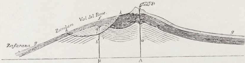
Fig. 97 Querschnitt durch die Val del Bove des Ätna (nach Ch. Lyell)
