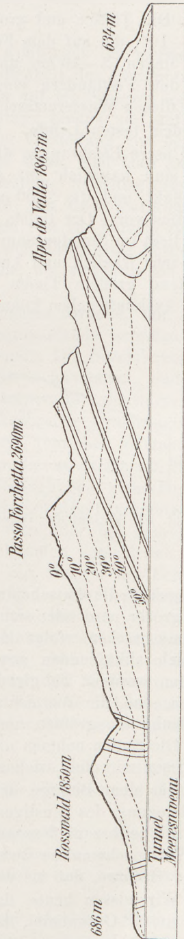
Fig. 9 Verlauf der Geoisothermen (gestrichelt) im Profil längs der Achse des Simplontunnels (nach G. Niethammer). Die vollaufgezogenen Linien zeigen die Lage der Schichtung.
