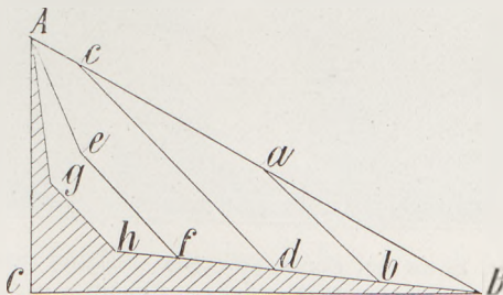
Fig. 262 Ausbildung der Gefällsterminante nach A. Philippson. A—B ursprüngliches Gefälle, AghB Endgefälle, AabB , AcdB , AefB Zwischenstadien, ab , cd , ef , gh Torrentpartien, Ae , Ay Kaskadepartien
