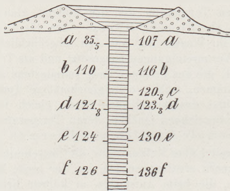
Fig. 304 Erklärung der Geysirtätigkeit (nach R. Bunsen). Die Zahlen links geben die gemessenen Temperaturen, die rechts sind die Siedetemperaturen bei dem entsprechenden Drucke. Bei c stimmen die beiden Werte überein und es erfolgt Verdampfung. An der vorspringenden Leiste scheint die Wärmezufuhr stattzufinden.
