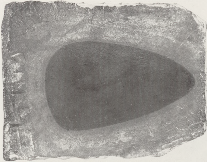
Fig. 232 Verfärbung durch Oxydation im Mergelkalke von Solnhofen
