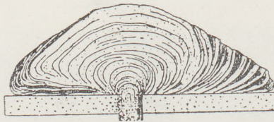
Fig. 53 Quellkuppe nach E. Reyer
