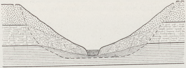
Fig. 246 Rutschungen an Talwänden in losem Terrain
