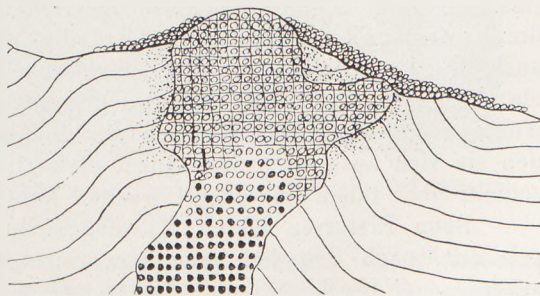
Fig. 38 Das kieselsäurereiche Tiefengestein tritt, von einem Kontakthofe umgeben, an die Oberfläche und liefert Verwitterungsprodukte. Das eisenreiche Magma der Tiefe ist noch nicht erstarrt.
