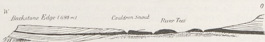
Fig. 35 Profil durch den großen Whin Sill, einen Lagergang (nach A. Geikie aus F. von Wolff)
