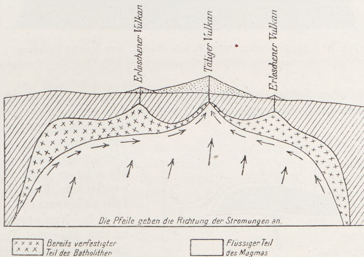
Fig. 30 Tätige und erloschene Vulkane über einem Batholithen (nach R. A. Daly aus F. von Wolf)
