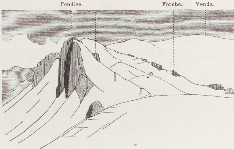
Fig. 112 Erodierte Radialgänge des Vulkanes Venda in den Euganeen (nach E. Reyer)
