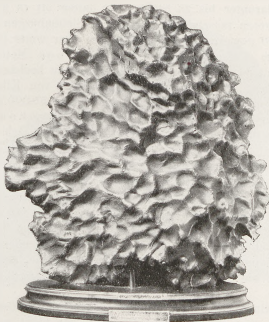
Fig. 15 Brustseite des Meteoreisens von Cabin Creek
