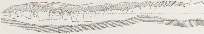
Fig. 332 Das Kalben von Gletschern in einem Fjorde Grönlands (nach A. Helland)
