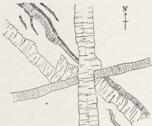
Fig. 34 Sich schneidende Gänge (nach A. Geikie aus F. von Wolff)
