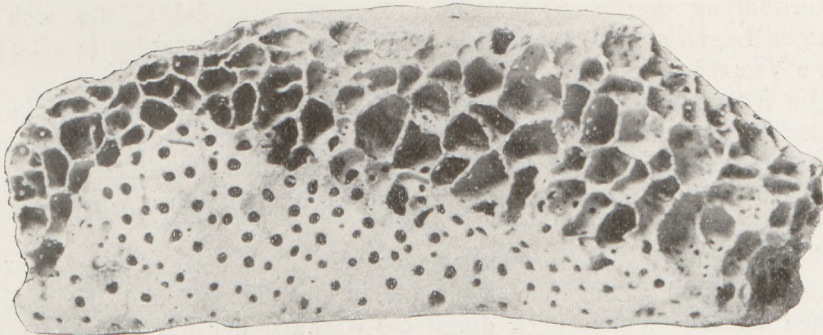
Fig. 242 Rezentes Strandgerölle, von Bohrschwämmen durchbohrt.
