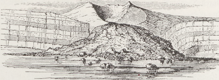
Fig. 43 Tertiärschichten, gegen den Eruptionsschlot einfallend, bei Auckland, Neuseeland (nach C. Heaphy aus P. Scrope)
