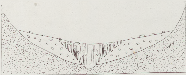
Fig. 252 Entstehung von Erdpyramiden (nach Ch. Lyell)
