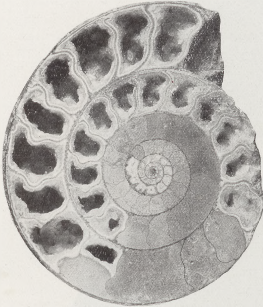
Fig. 452 Durchschnitt durch einen Ammoniten, dessen Luftkammern zum Teil mit Kalkspatkristallen ausgekleidet, zum Teil von Sediment erfüllt sind.
