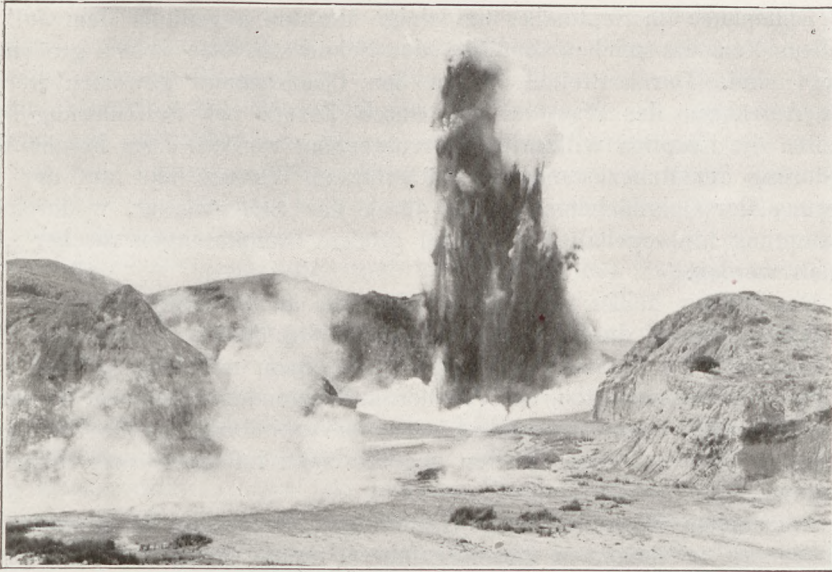
Fig. 307 Waimango Geysir bei Rotorua, Neuseeland, im Höhepunkte der Eruption
