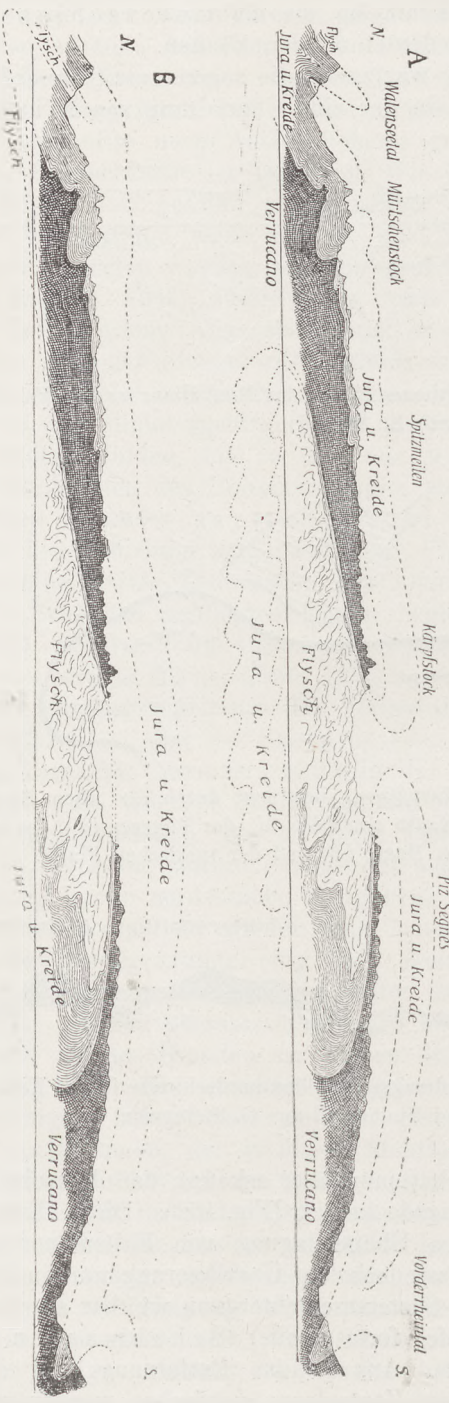
Fig. 181 Querschnitt durch die Glarner Überfaltungsregion nach der Deutung als Doppelfalte nach A. Heim Fig. 182 Dasselbe Profil nach der neuen Auffassung als Überfaltungsdecke nach M. Lugeon (beide aus G. Steinmann)
