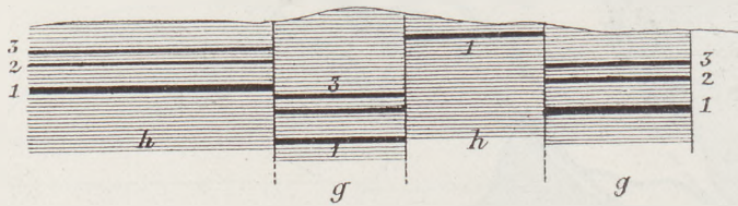
Fig. 137 An vertikalen Brüchen abgesunkene Schollen. g, g Gräben; h, h Horste (nach F. Löwl)
