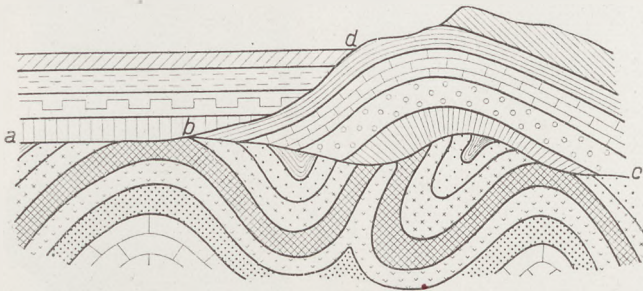
Fig. 162 Wiederholte Diskordanz. Ein konkordantes, gefaltetes Schichtsystem wurde nach der Linie a-b-c abgetragen und mit den diskordant darüber abgelagerten, wieder untereinander konkordanten Schichten neuerdings gefaltet und auf der neuen Abtragungsfäche a-b-d lagerten sich wieder diskordant jüngere, untereinander konkordante Schichten ab.
