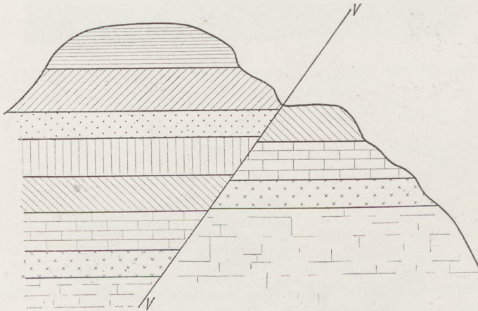
Fig. 133 Unterdrückung von Schichtgliedern (3 und 4 von oben) im Profile durch eine Verwerfung V—V
