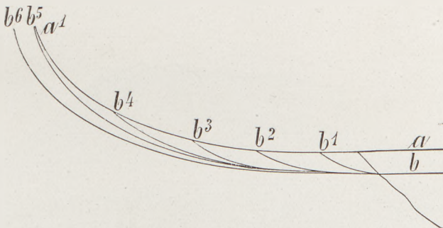
Fig. 277 Der Fluß hat in a-a^1 seine Endkurve erreicht. Durch Verlegung der Erosionsbasis von a nach b wird die Erosion belebt und er nimmt die Kurven a^1 b^1 b , a^1 b^2 b , a^1 b^3 b , a^1 b^4 b , b^5 b ein. Seine Endkurve erreicht er erst in b^6 b .
