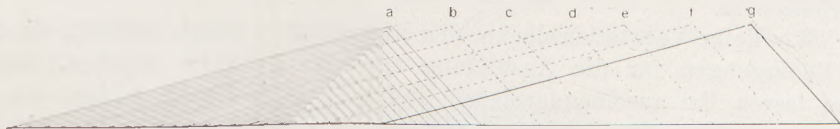
Fig. 351 Schematische Darstellung des Baues und des Wanderns einer Düne, a—g aufeinanderfolgende Lagen des Kammes
