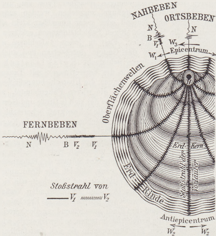
Fig. 184 Schematische Darstellung der Fortpflanzung der seismischen Wellen und ihres Erscheinens im Seismogramm (nach A. Sieberg). H Hypozentrum, V_1 die ersten, V_2 die zweiten Vorläufer, B lange Wellen des Hauptbebens, N Nahbeben, W_1 , W_2 , W_3 Oberflächenwellen erster, zweiter, dritter Ordnung
