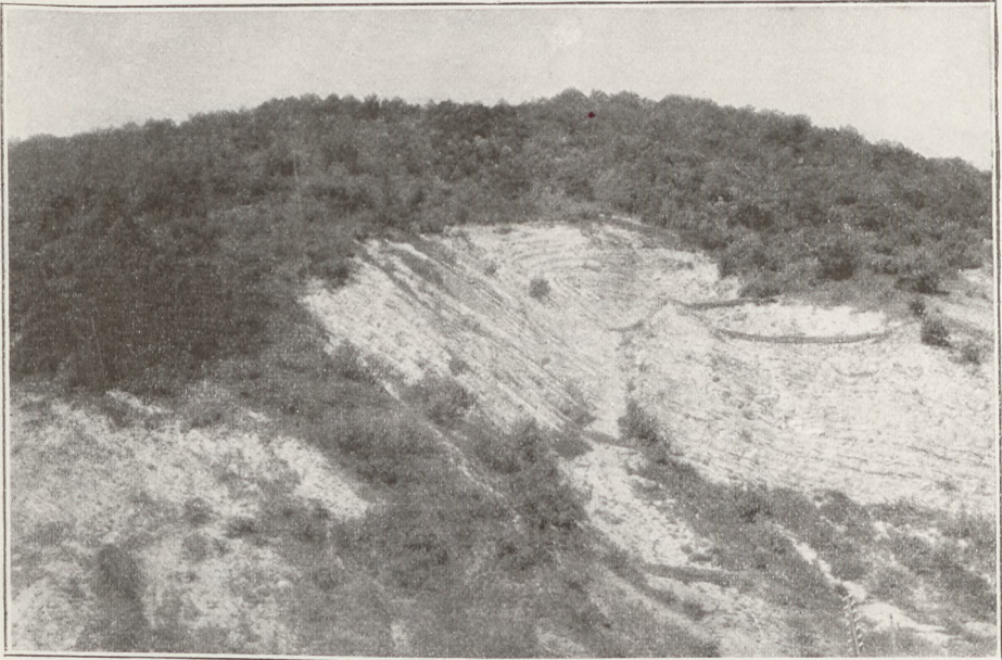
Fig. 149 Liegende Falte am Leopoldsberge bei Wien (phot. F. X. Schaffer)
