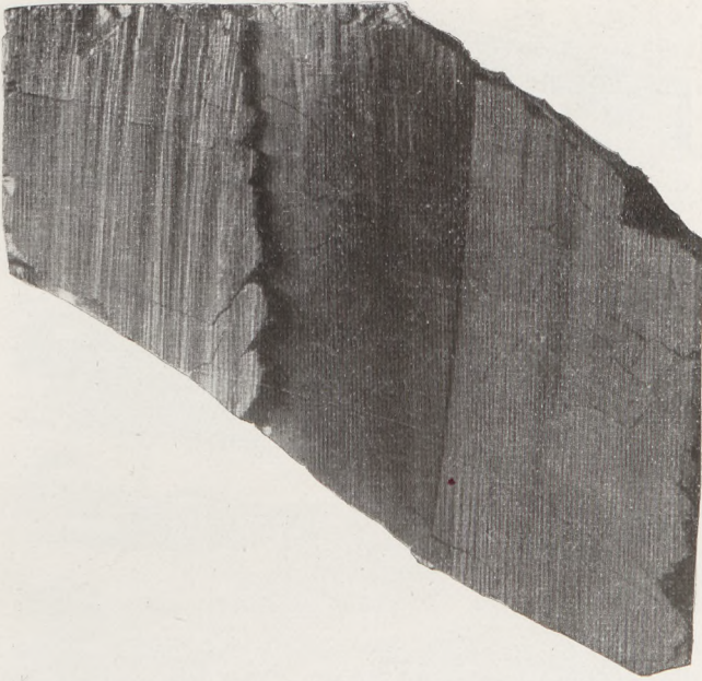
Fig. 126 Braunkohle mit Harnisch und Riefen von Fohnsdorf
