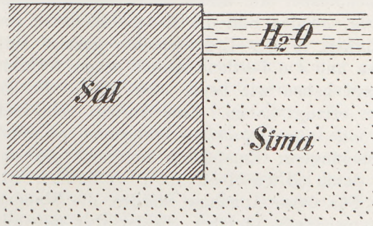
Fig. 7 Schematischer Querschnitt durch einen Kontinentalrand nach A. Wegener. Zeigt das Schwimmen der Kontinentschollen (Sal) auf dem Simamantel und ihr Emporragen über die Meeresfläche.
