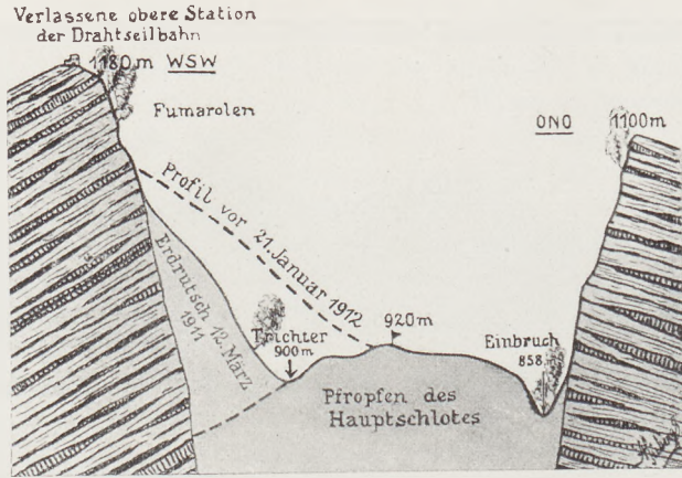
Fig. 89 Schematischer Schnitt durch den Vesuvkrater (nach den Aufnahmen von A. Malladra aus A. Sieberg)
