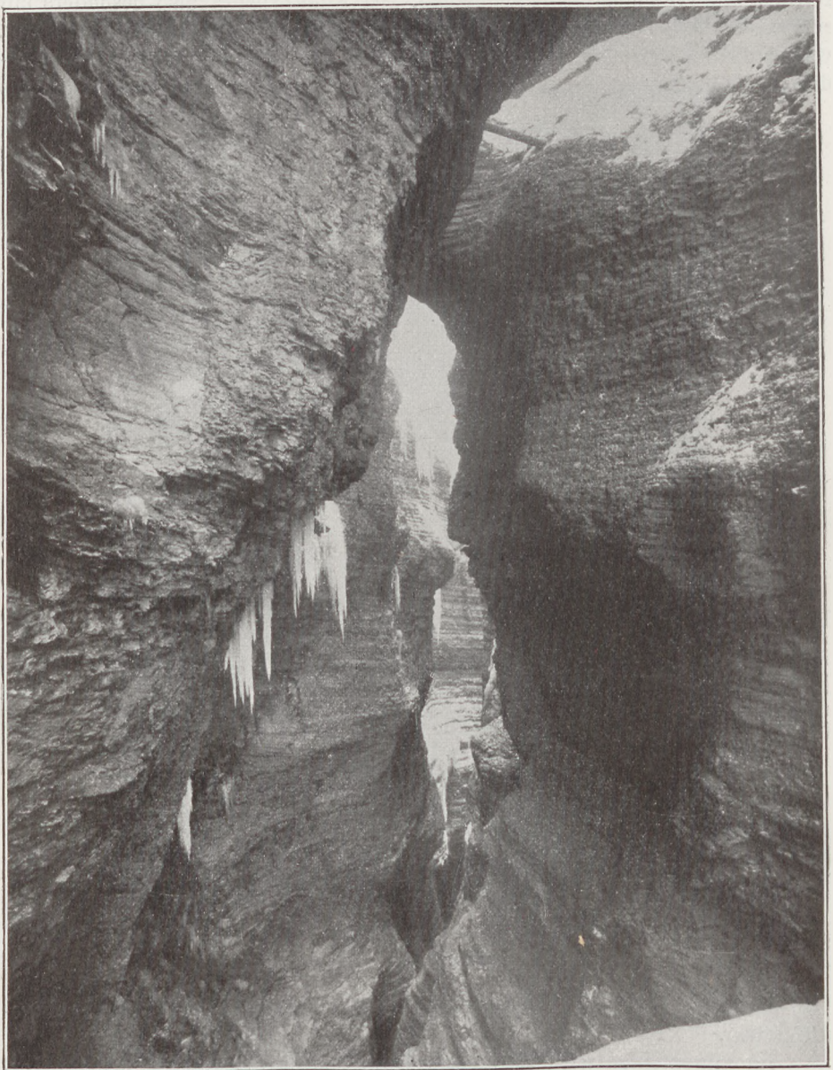
Fig. 268 Schlucht der Fersina bei Ponte Alto unweit Trient in dünngeschichteten Kalken (nach einer Aufnahme von G. B. Unterveger, Trient)
