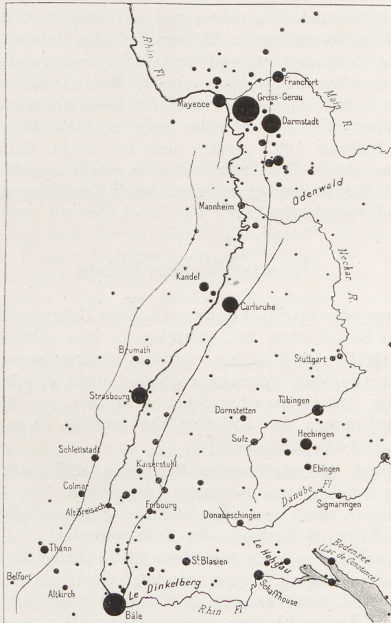
Fig. 191 Verteilung der Erdbeben im Mittelrheingraben (nach F. de Montessus de Ballore)
