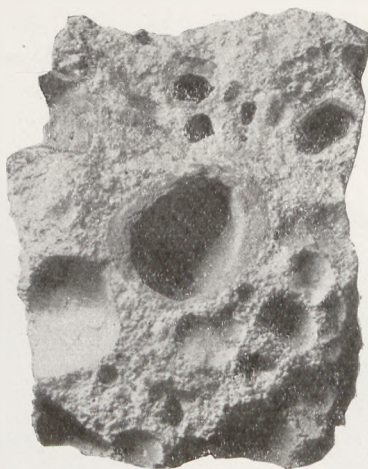
Fig. 409 Hohle Gerölle
