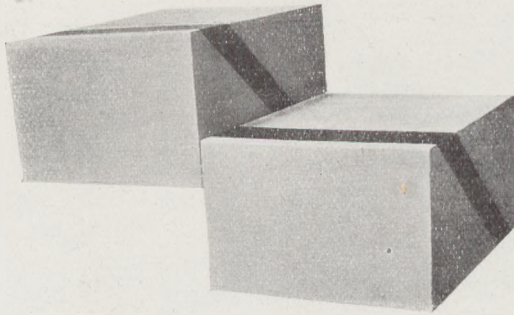
Fig. 129 Querwerfung einer Schicht (schwarz angelegt)
