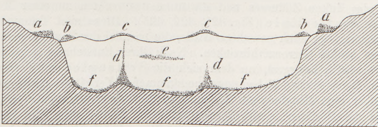
Fig. 325 Querschnitt durch einen Gletscher, a Ufermoräne, b Seitenmoräne, c Mittelmoräne, d Scheide- (Einscharungs-) moräne, e Innenmoräne, f Grundmoräne
