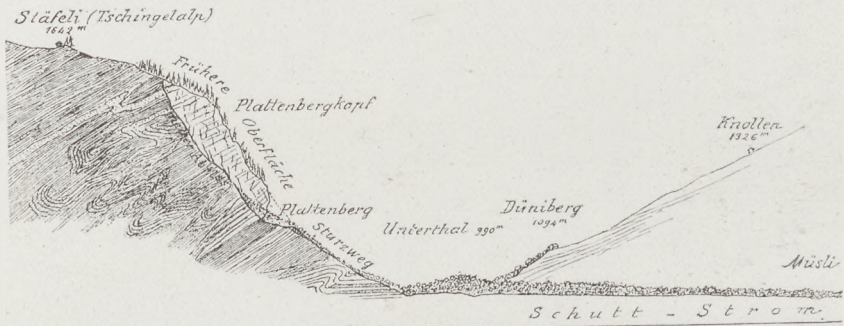
Fig. 247 Profil des Bergsturzes von Elm 1881 (nach A. Heim)
