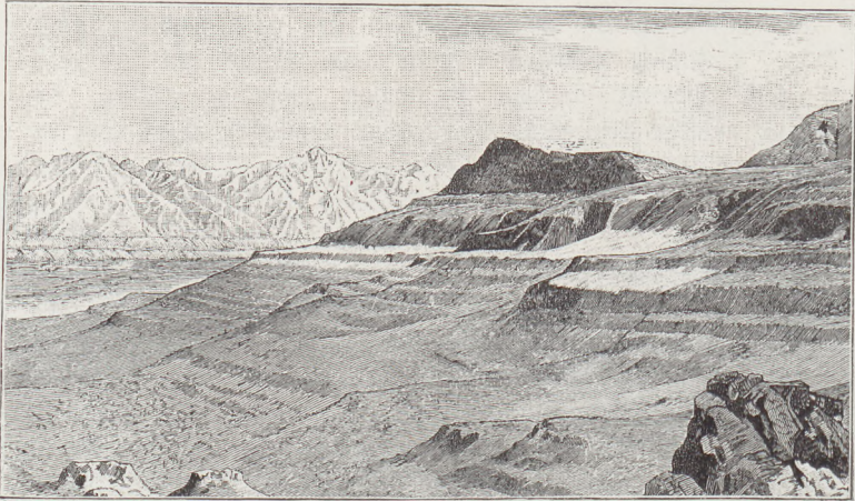
Fig. 319 Strandterrassen am einstigen Bonneville-See, Utah, Nordamerika (nach G. K. Gilbert)
