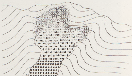
Fig. 37 Durch Abtragung gelangt das metamorphosierte Gestein an die Oberfläche und läßt den Stock in der Tiefe vermuten, in dem bei fortschreitender Erstarrung eine Sonderung der Gemengteile nach dem spezifischen Gewichte erfolgt.
