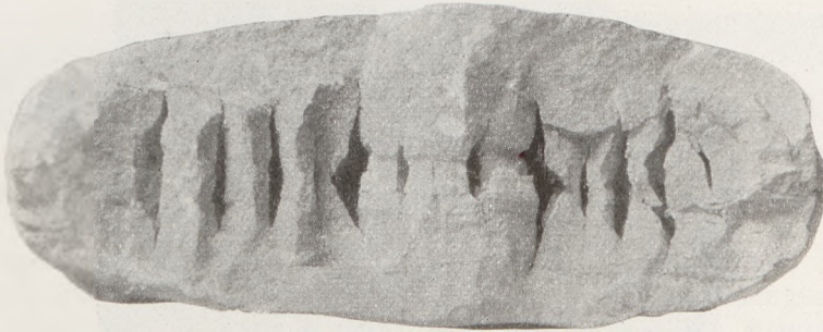
Fig. 413 Septarie aus Kalkmergel
