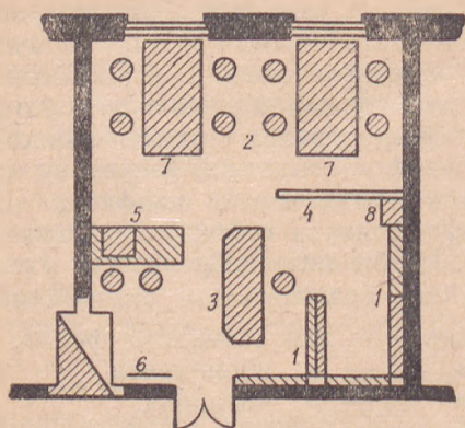
Рис. 1-а. Расположение библиотеки в комнате площ. 25 кв. м. Вариант расстановки при дальнейшем росте книжного фонда и увеличении количества книжных стеллажей (сравни с рис. 1)
