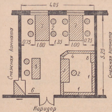
Рис. 1. Расположение библиотеки с книжным фондом в 1600 томов в комнате площ. 25 кв. м. Оборудование: 1 — книжные стеллажи, 2 — стулья, 3 — стол выдачи, 4 — барьер, 5 — каталожный шкафчик на століке, 6 — книжные витрины, 7 — столы для чтения на 4 места (двухсторонние), 8 — шкаф для документов
