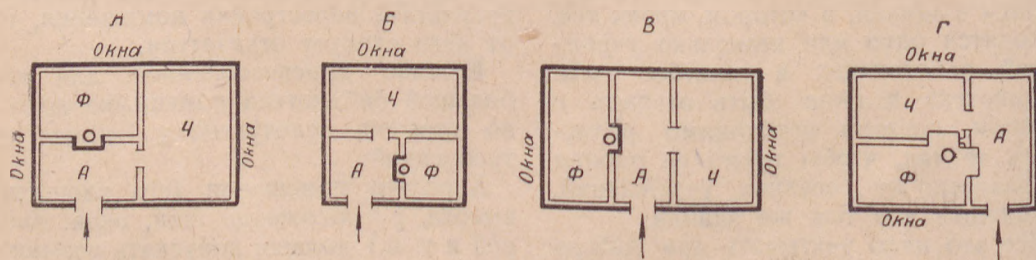
Схема общей организации сельской библиотеки в зависимости от условий помещения
