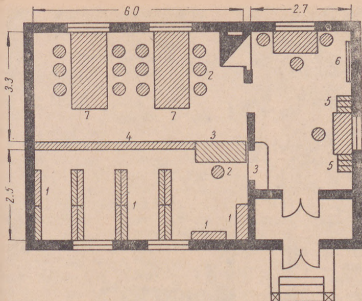
Рис. 5. Расположение библиотеки в пятистенной избе. Оборудование: 1 — книжные стеллажи, 2 — стулья, 3 — стол выдачи, 4 — барьер, 5 — каталожные шкафчики со столиком, 6 — витрина, 7 — столы для чтения двухсторонние, шестиместные
