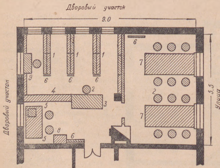
Рис. 4-б. Расположение библиотеки в двух комнатах общей площадью в 48,5 кв. м. Оборудование: 1 — книжные стеллажи, 2 — стулья, 3 — стол выдачи, 4 — барьер, 5 — каталожный шкафчик со столом, 6 — книжные витрины, 7 — столы для чтения двухсторонние, шестиместные, 8 — шкаф для документов, 9 — рабочий столик
