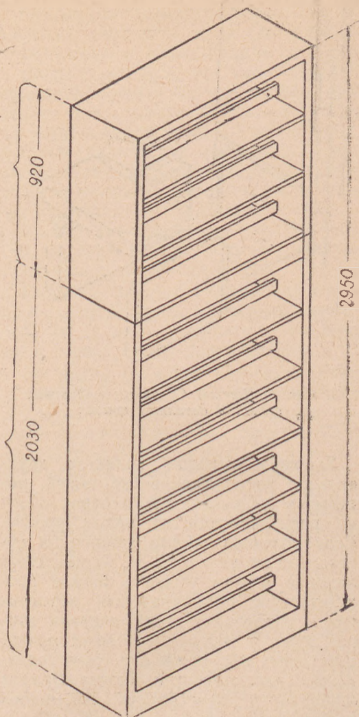
Рис. 10. Пример временного образования составного книжного стеллажа с повышенным количеством полок из обычного шестиполочного стеллажа и дополнительных трех полок
