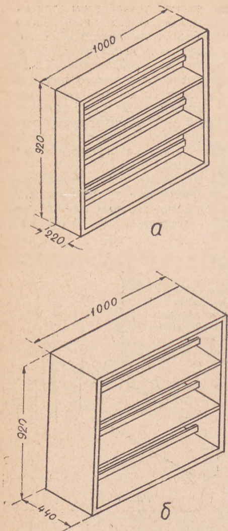
Рис. 9. Элементы для наращивания книжного стеллажа дополнительными полками: а) одно-стороннего, б) двустороннего
