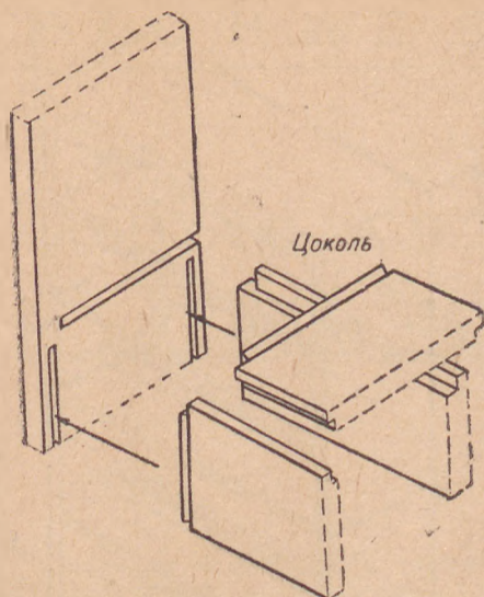
Рис. 6. Цоколь. Сопряжение боковых стенок с деталями цоколя
