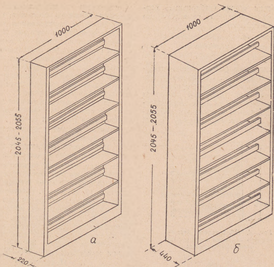
Рис. 3. Общий вид секции книжного стеллажа: а) одностороннего, б) двустороннего
