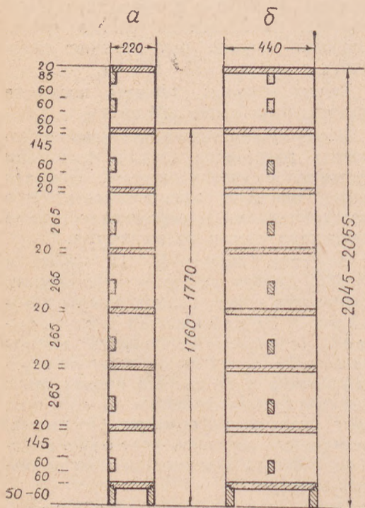
Рис. 2. Разрез книжного стеллажа: а) одностороннего, б) двустороннего
