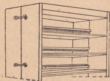
Рис. 4. Образование двустороннего стеллажа соединением двух односторонних
