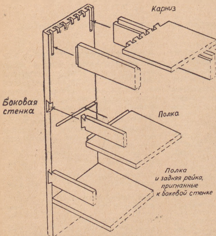
Рис. 5. Сопряжение боковых стенок с полками и деталями верхней части (карниза)
