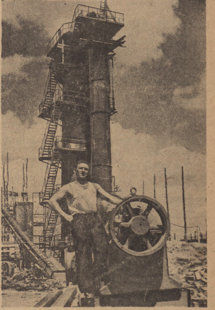
Budowa nowoczesnej cukrowni w Sokolowie Podlaskim. Na zdjęciu: brygadziści produkujący na budowie zespołu — Roman Wojtaszek. W głębi — piec zmontowany przez jego brygadę. Foto CAF
