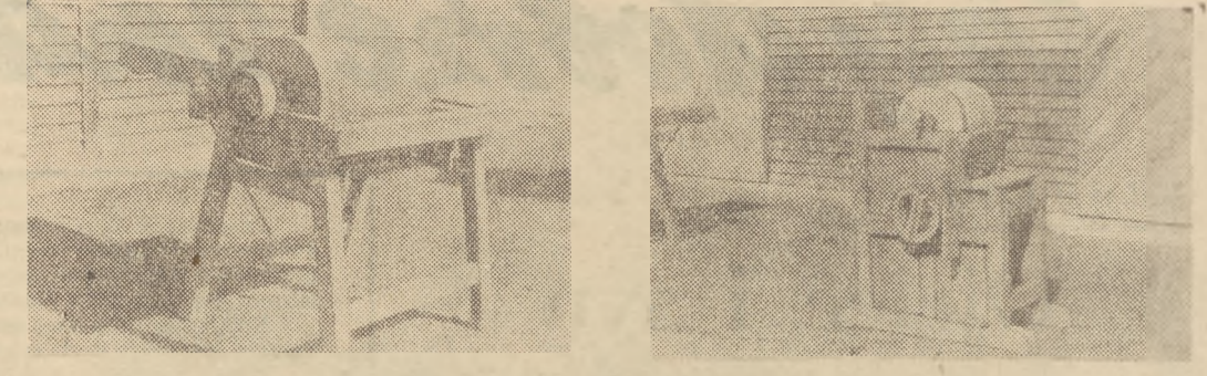
Młocarka do sorga miotłkowego.
