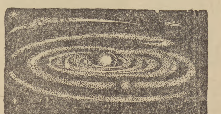
Powstanie układu słonecznego według Laplace'a. Od wirującej i zagęszczającej się mgławicy oddzieliły się pierścienie, które stopniowo skupiały się w kuliste zagęszczenia — planety. Z materii pozostałej w centrum powstało Słońce.
