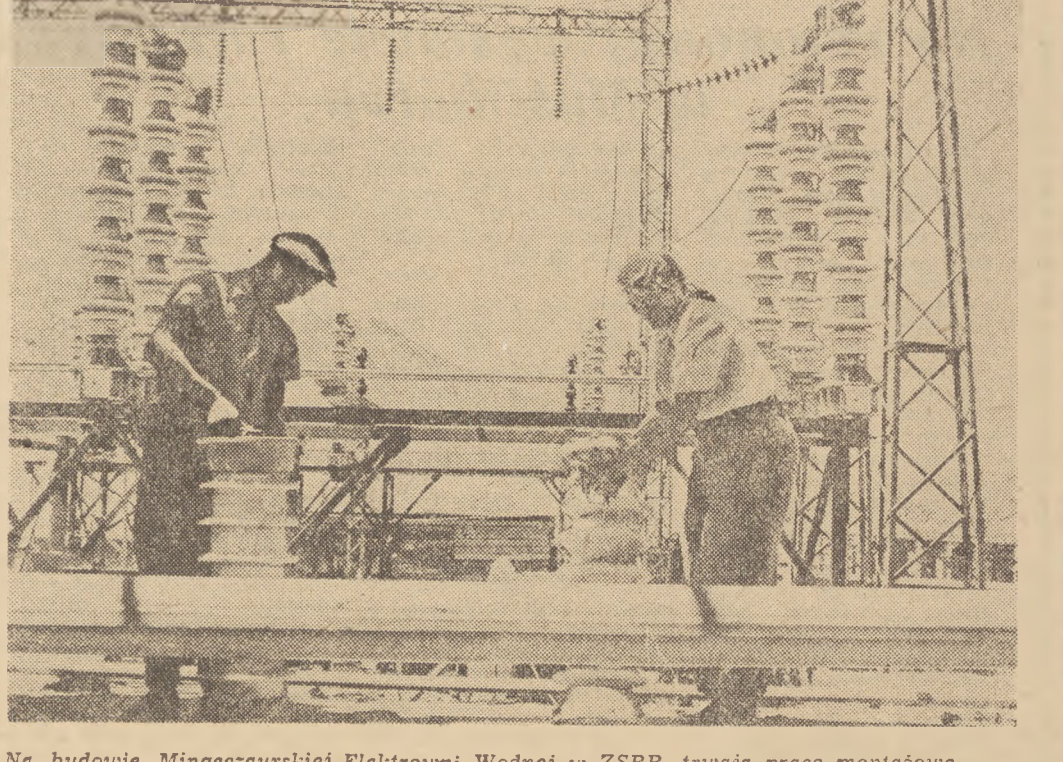
Na budowie Mingcaurskiej Elektrowni Wodnej w ZSRR trwają prace montażowe. Na zdjęciu: J. Mamulin i T. Kustowa przy montażu transformatora. Fot. CAF
