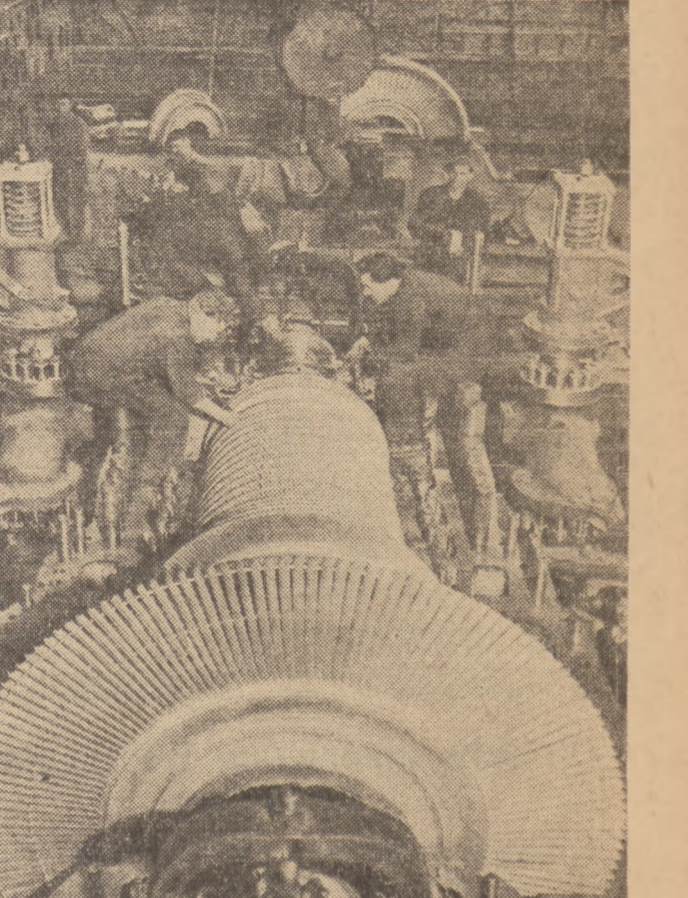
Prace montażowe związane z uruchomieniem elektrociepłowni żerańskiej szybko postępują naprzód. Na zdjęciu: brigada Stefana Banasza sprząda pod kierunkiem radzieckiego specjalisty inż. Amielina centrumie wirnika turbiny. Foto CAF — Baranowski
