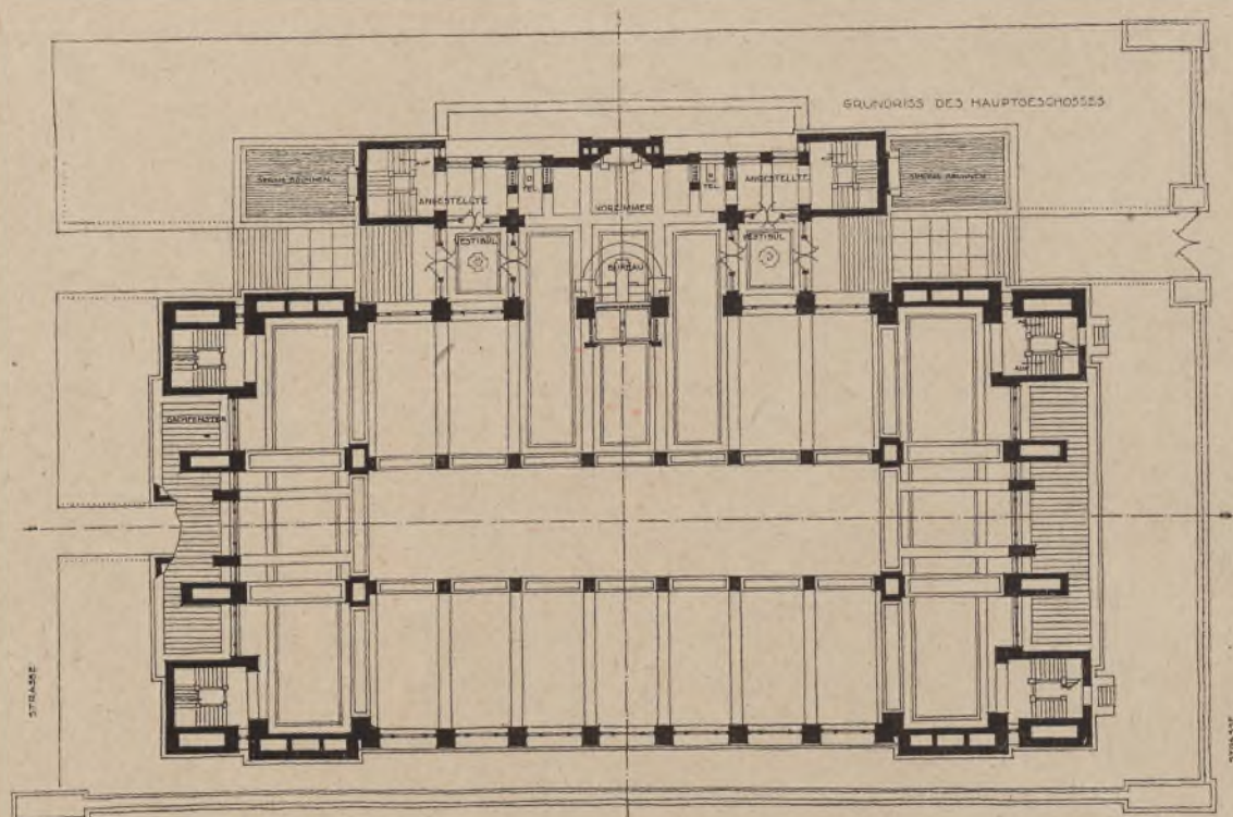
ARCHITEKT: F. L. WRIGHT, VERWALTUNGSGEBAUDE CHICAGO. HAUPTGESCHOSSGRUNDRISS
