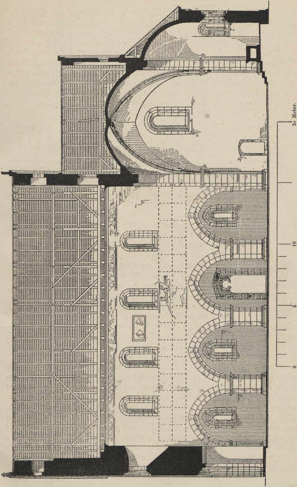
Fig. 5. Längschnitt der St. Nicolaikirche zu Dippoldiswalde.
