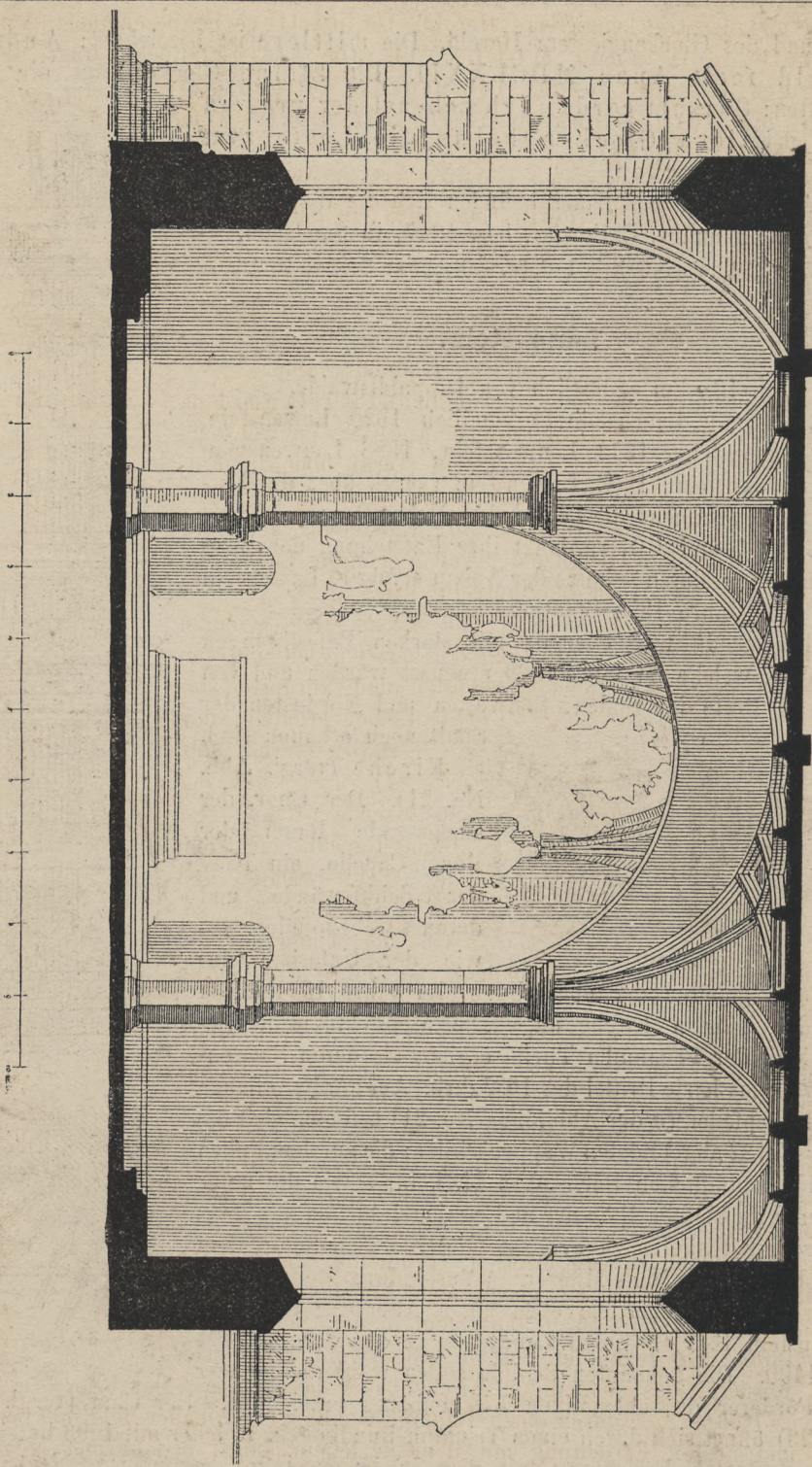
Fig. 23. Querschnitt der Kirche zu Lauenstein, nach dem Altar zu gesehen.
