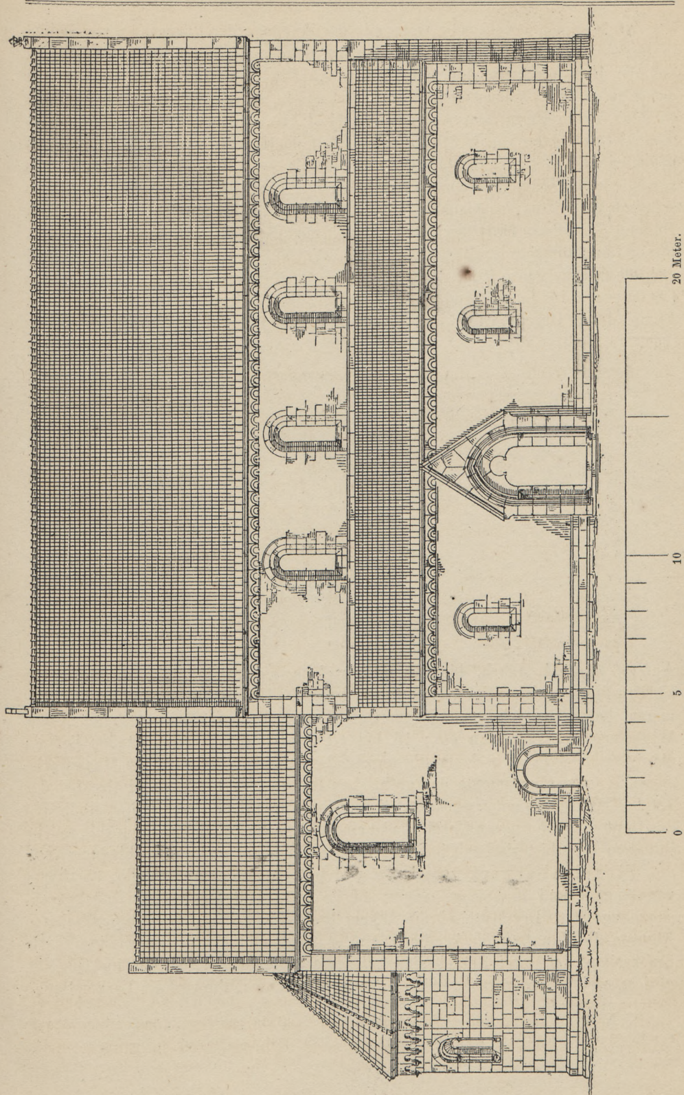
Fig. 8. Nordfaçade der St. Nikolaikirche zu Dippoldiswalde.
