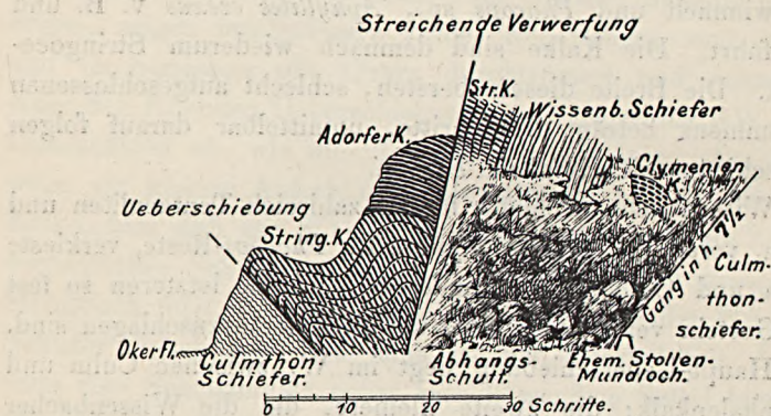
Profil der Devonschichten
