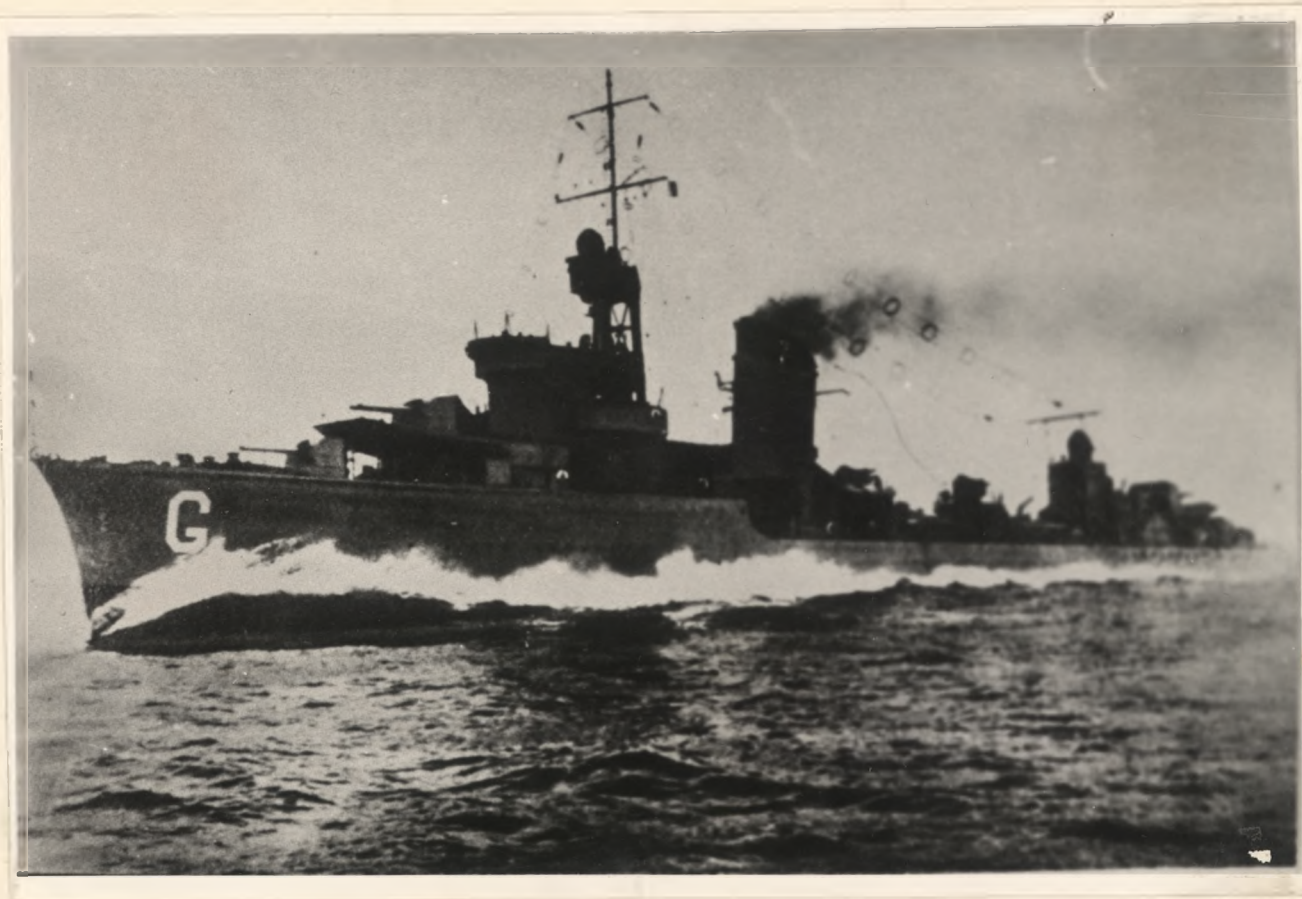
Zdjęcie "GROMA" wykonane w czasie próby szybkości na pełnym morzu. Zdjęcie to firma SAMUEL WHITE przez wiele lat zamieszczała w rocznikach flot, reklamując nim budowane przez siebie okręty.
