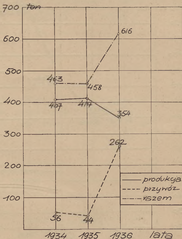
Rys. 9. Tiosiarczan sodu.
