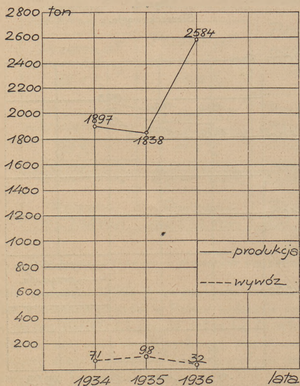
Rys. 8. Siarczek sodu.
