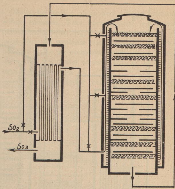
Rys. 2. Aparat półkowy.
