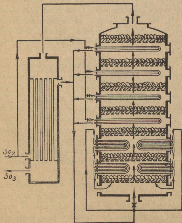
Rys. 4. Aparat Favser'a z rurami chłodzącymi.
