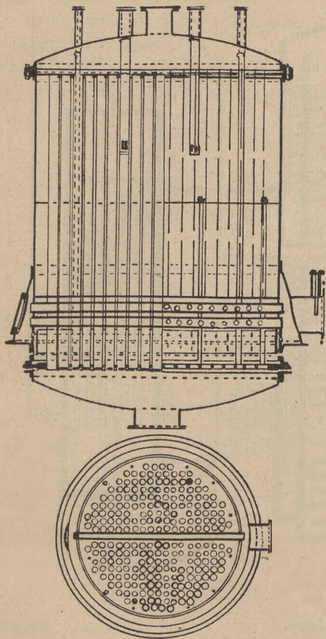
Rys. 1. Aparat rurowy.
