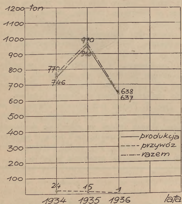
Rys. 12. Aluny.
