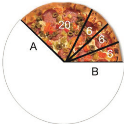
Rys. 1. Przykład końcowej partii gry
