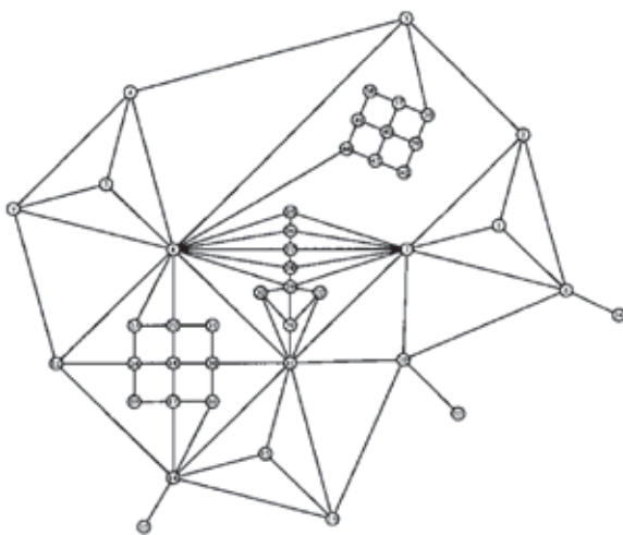
Rys. 2. Zwycięzca z roku 1994 w kategorii grafów planarnych
