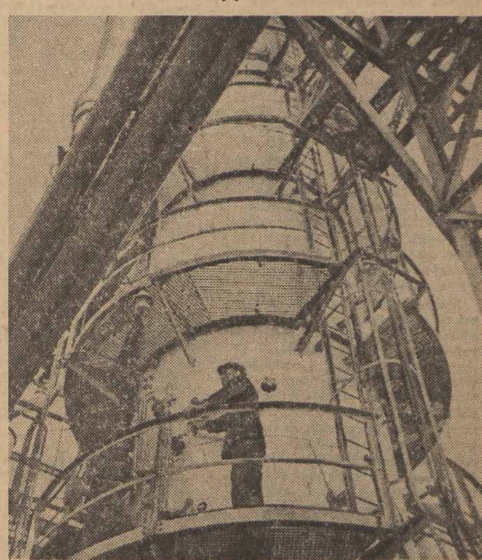
W Trzebini dobiega końca budowa nowoczesnego zakładu przemysłowego dla przeróbki ropy naftowej Uruchomienie nowego obiektu pozwoli na 4-krotnie zwiększenie przeróbki ropy w tym okręgu. Na zdjęciu: fragment budowy destylatorni. Foto CAF — Tymusk
