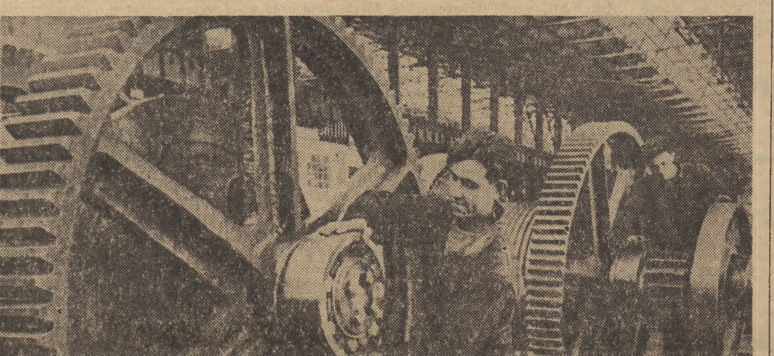
Fabryki radzieckie dostarczają budowniczym wielkich budowli komunizmu wspaniały sprzęt. Brygada monterska oddziału koparek w Nowoakramatorskiej Fabryce im. Stalina wykonuje plan produkcyjny w 200 - 250 procentach. Na zdjęciu: ślusarze-montarze S. Kosińskianin (od lewej) i I. Terechow przy montowaniu głównych łożysk do koparek kroczących.
